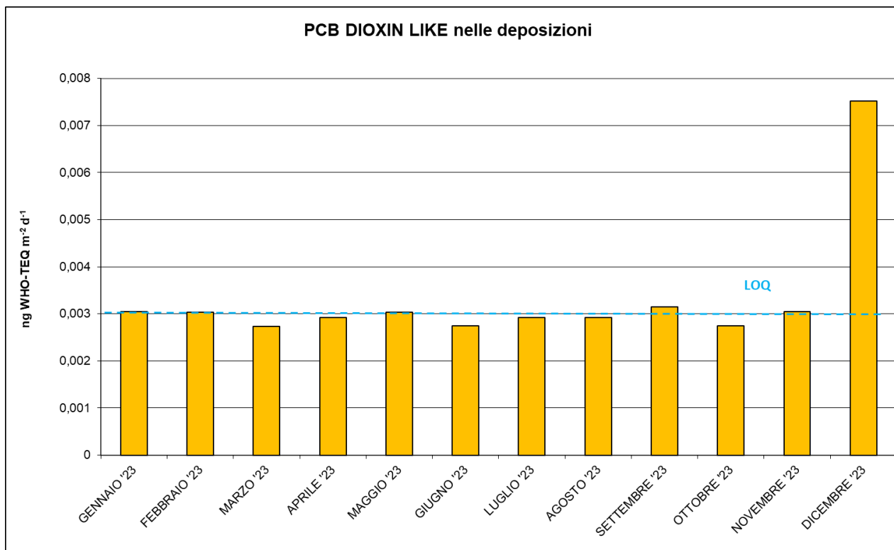
Figura 46 - Concentrazione di PCB DIOXIN LIKE nelle deposizioni mensili anno 2023
