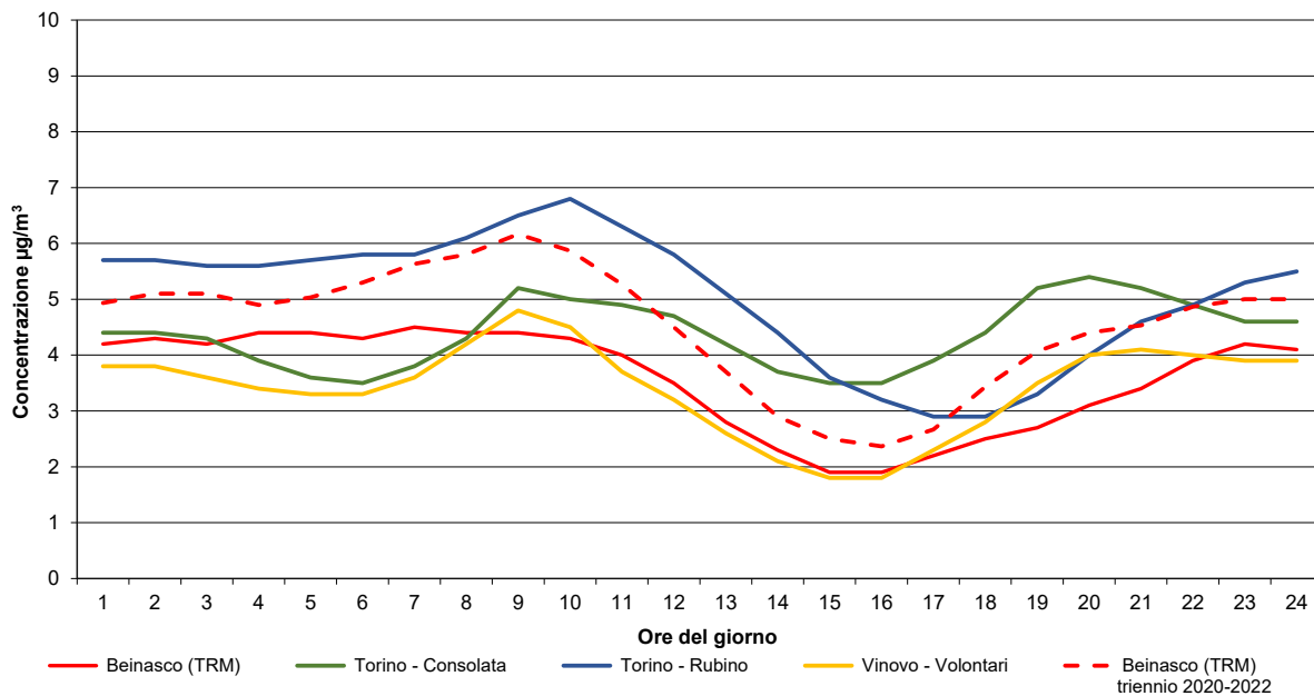
Figura 15 - Andamento medio delle concentrazioni orarie di Toluene (giorno medio)
