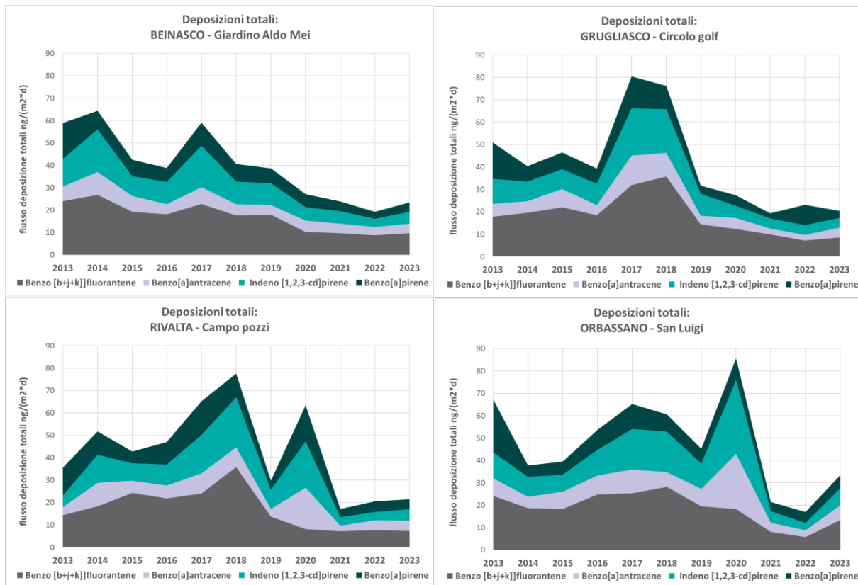
Figura 29 - andamenti cumulati di IPA nei siti di misura provinciali – periodo 2013-2023
