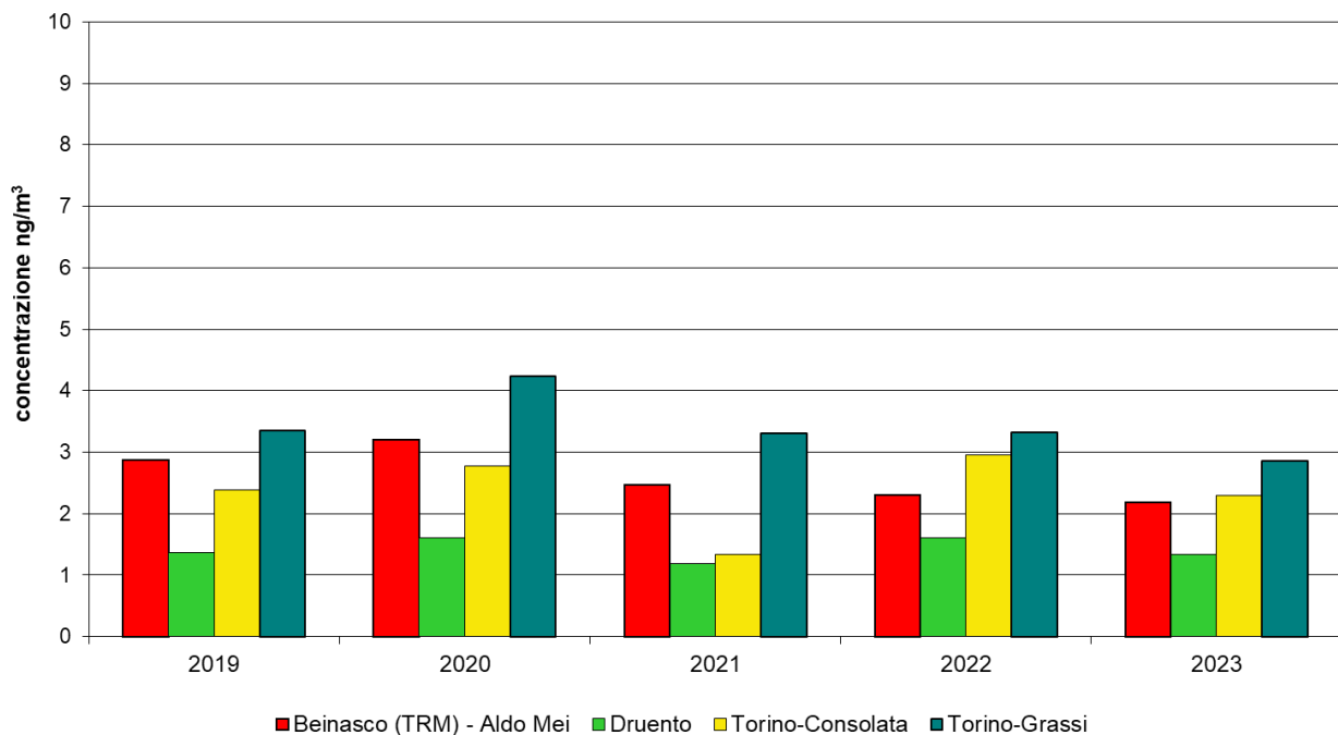
Figura 19 - Concentrazione degli IPA rilevati nel PM10 presso la stazione TRM Beinasco e in altre stazioni di confronto nel periodo 2019 - 2023
