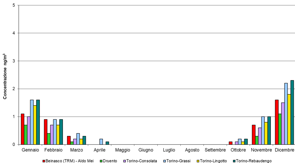
Figura 21 - Concentrazione di Benzo(a)Pirene nel PM10, andamento mensile nel 2023
