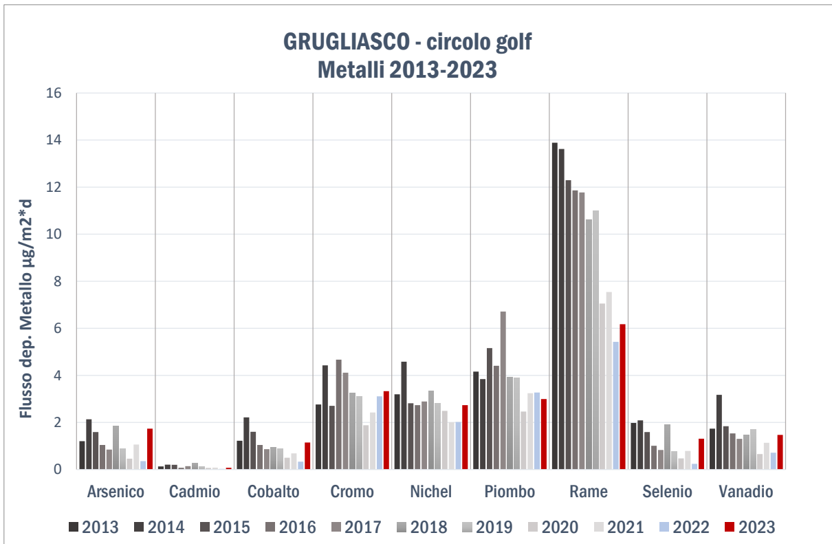
Figura 40 - Deposizioni metalli 2013-2023 nel sito di Grugliasco – circolo golf
