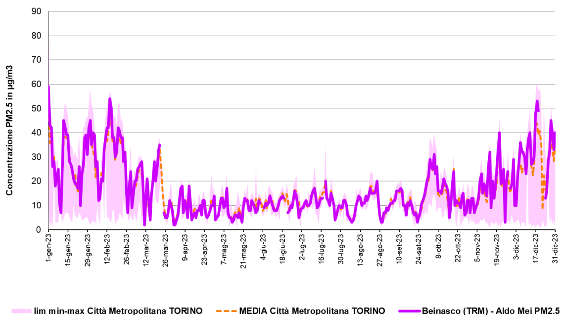
Figura 13 - PM2.5: Indici statistici anno 2023
