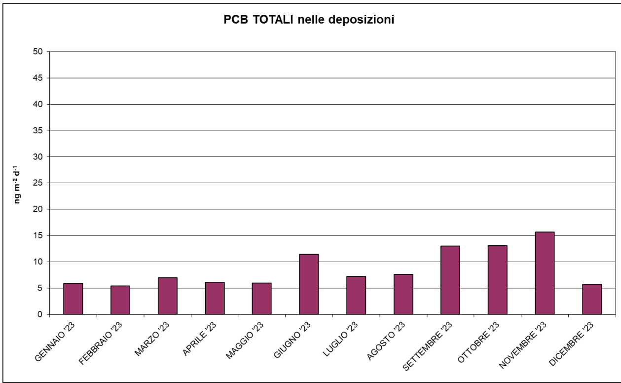
Figura 47 - Concentrazione di PCB TOTALI nelle deposizioni mensili anno 2023
