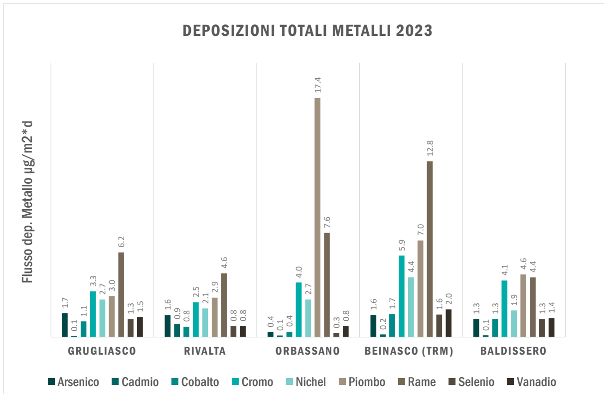
Figura 37 - Flusso deposizioni totali metalli nel 2023 per le stazioni della Città Metropolitana di Torino
