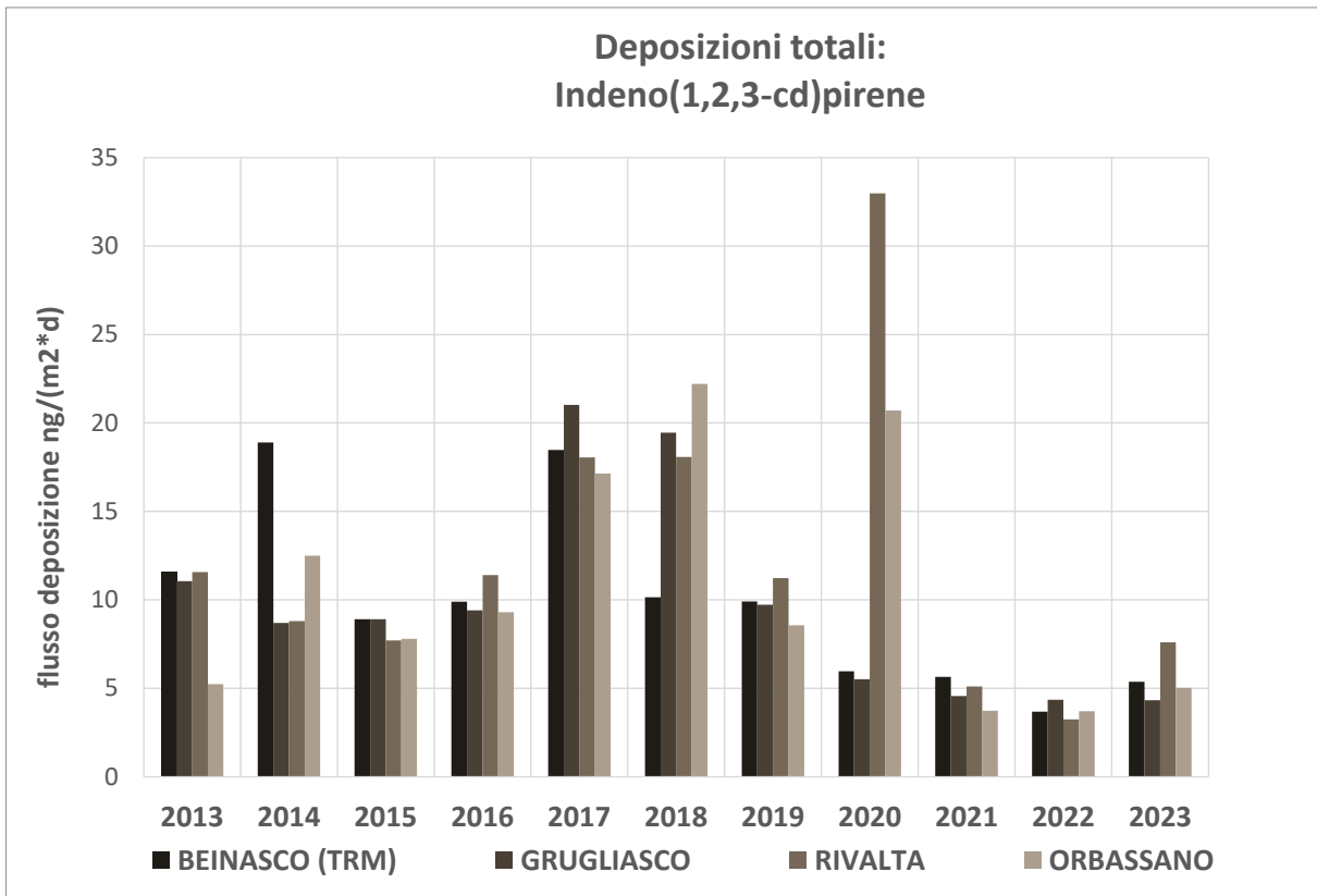
Figura 33 - Indeno(1,2,3-cd)pirene nelle deposizioni: confronto andamento 2013-2023
