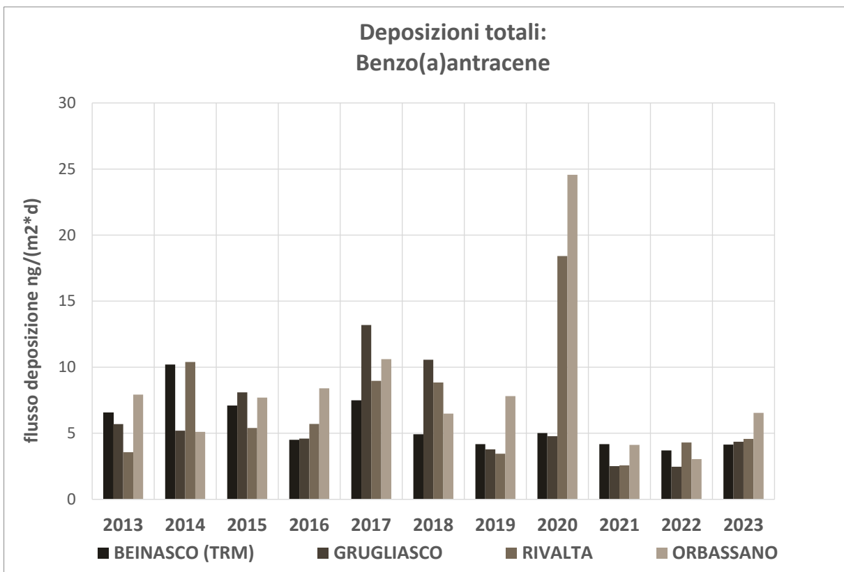
Figura 34 - Benzo(a)antracene nelle deposizioni: confronto andamento 2013-2023
