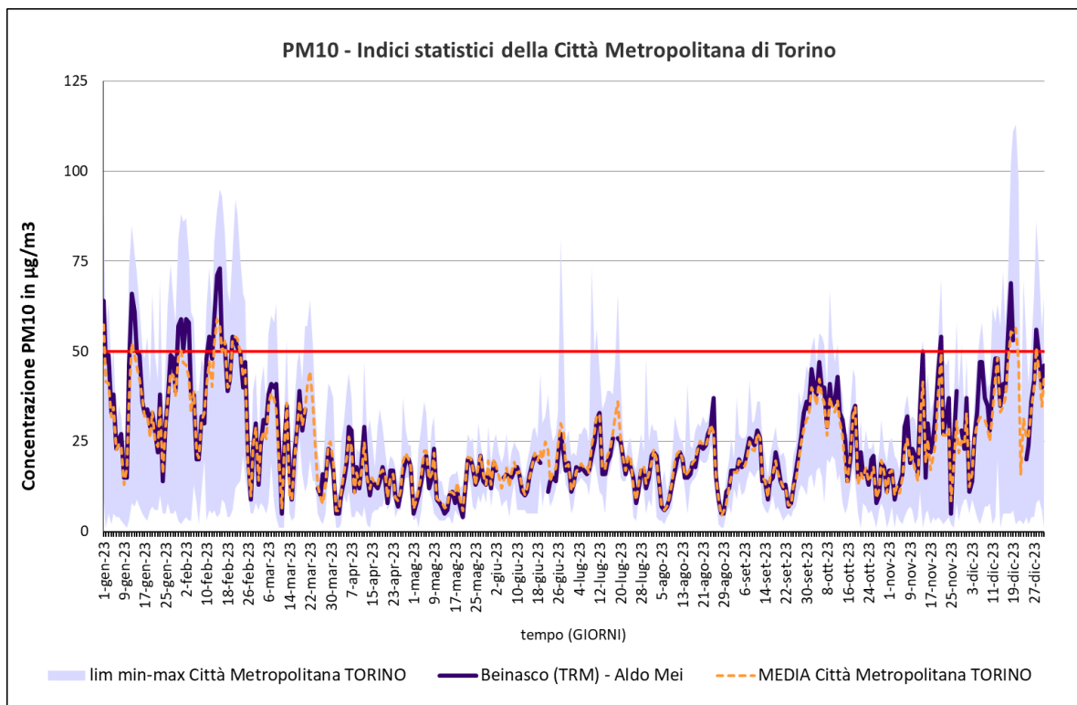
Figura 9 - PM10: Indici statistici anno 2023
