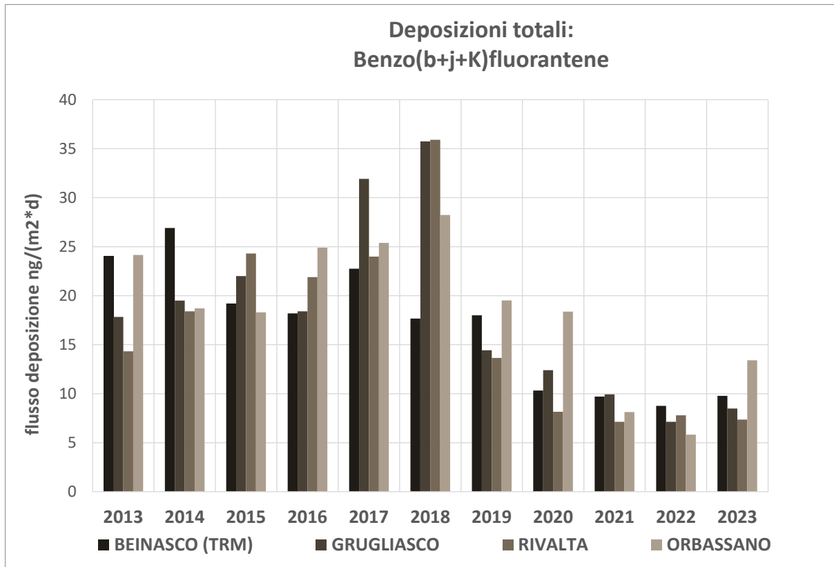
Figura 35 - Benzo(b+j+k)fluorantene nelle deposizioni: confronto andamento 2013-2023
