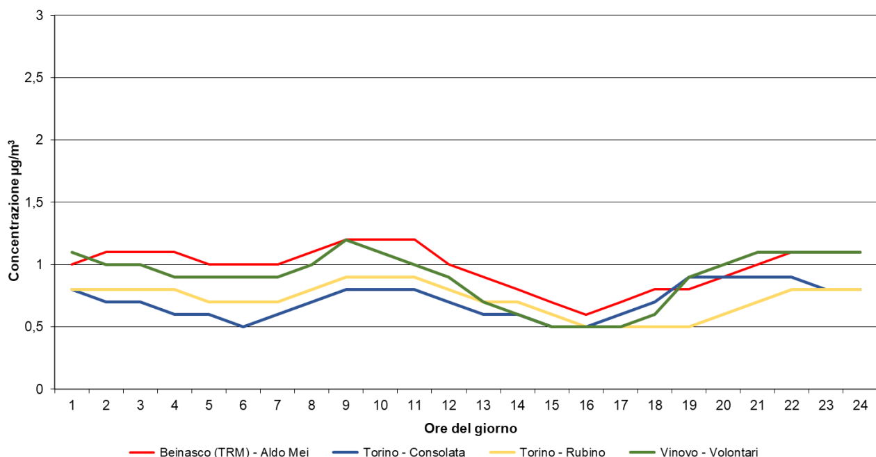
BENZENE - GIORNO MEDIO: confronto stazione TRM Beinasco con altre stazioni della Rete Regionale di Rilevamento della Qualità dell'Aria - Anno 2023
