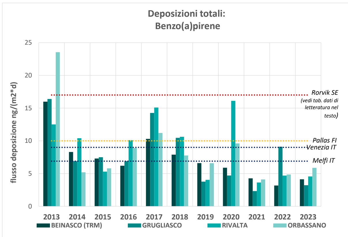
Figura 32 - Benzo(a)Pirene nelle deposizioni: confronto andamento 2013-2023
