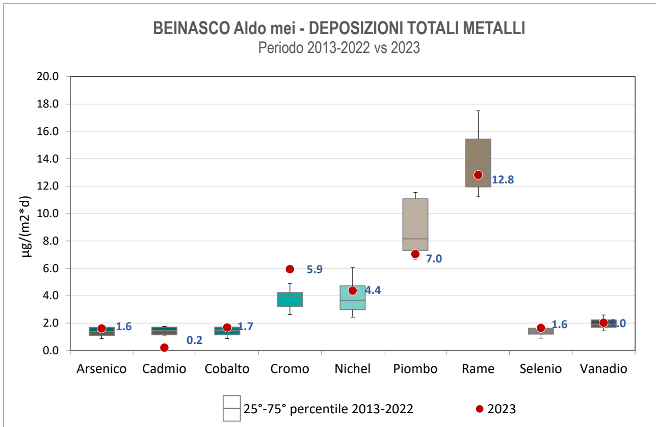
Figura 36 - Metalli nelle deposizioni: confronto periodo 2013-2022 e anno 2023 per la stazione di Beinasco Aldo Mei
