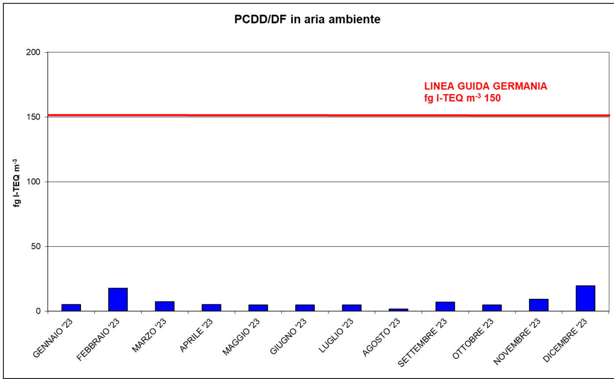
Figura 23 - Concentrazioni di PCDD e PCDF in aria ambiente anno 2023
