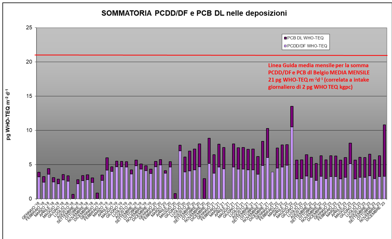
Figura 48 - Andamento sommatoria PCDD/DF + PCB dioxin like nelle deposizioni mensili dal 2018
