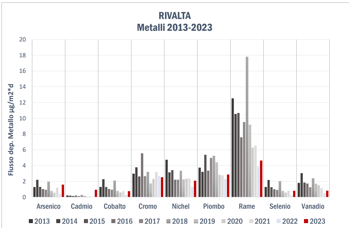
Figura 41 - Deposizioni metalli 2013-2023 nel sito di Rivalta – campo pozzi
