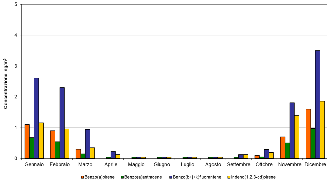
Figura 20 – Concentrazione degli IPA rilevati nel PM10 presso la stazione TRM Beinasco – Aldo Mei nel 2023
