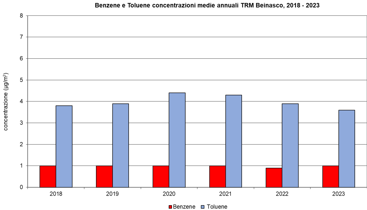
Figura 18 – Andamento concentrazioni medie annuali del benzene e del toluene della stazione TRM di Beinasco – Anni 2018 – 2023
