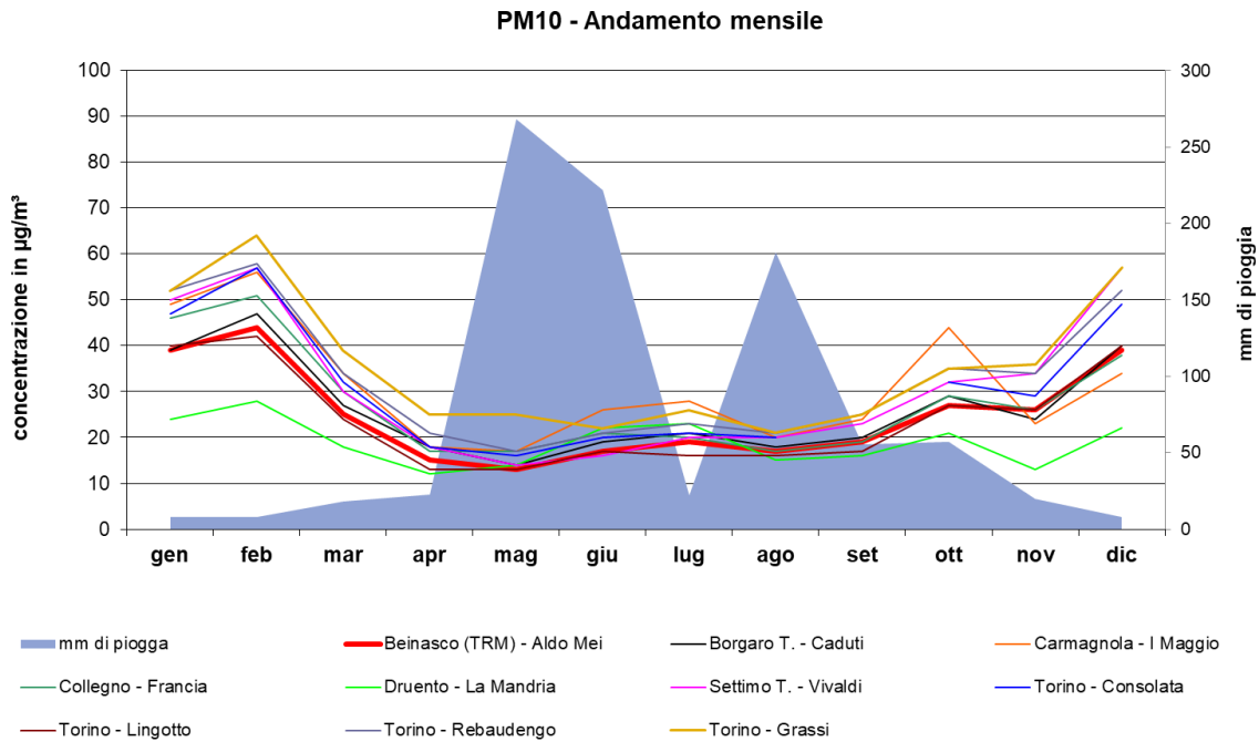
Figura 8 - PM10: Media mensile anno 2023
