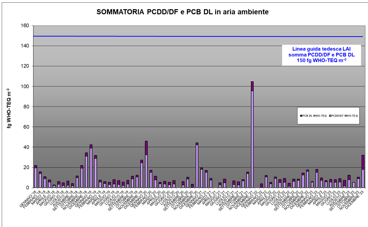
Figura 26 – Andamento sommatoria PCDD/DF + PCB dioxin like in aria ambiente dal 2018
