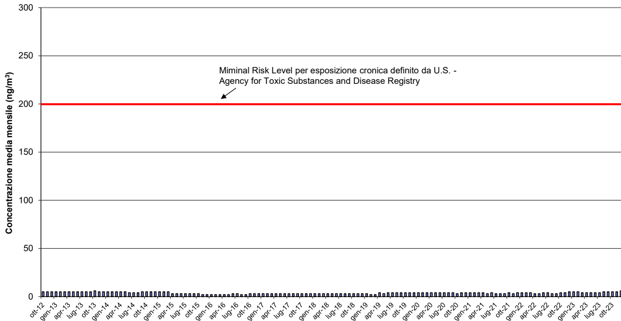
Figura 22 - Andamento delle concentrazioni mensili di mercurio nella stazione di Beinasco Aldo Mei dal 2012 al 2023
