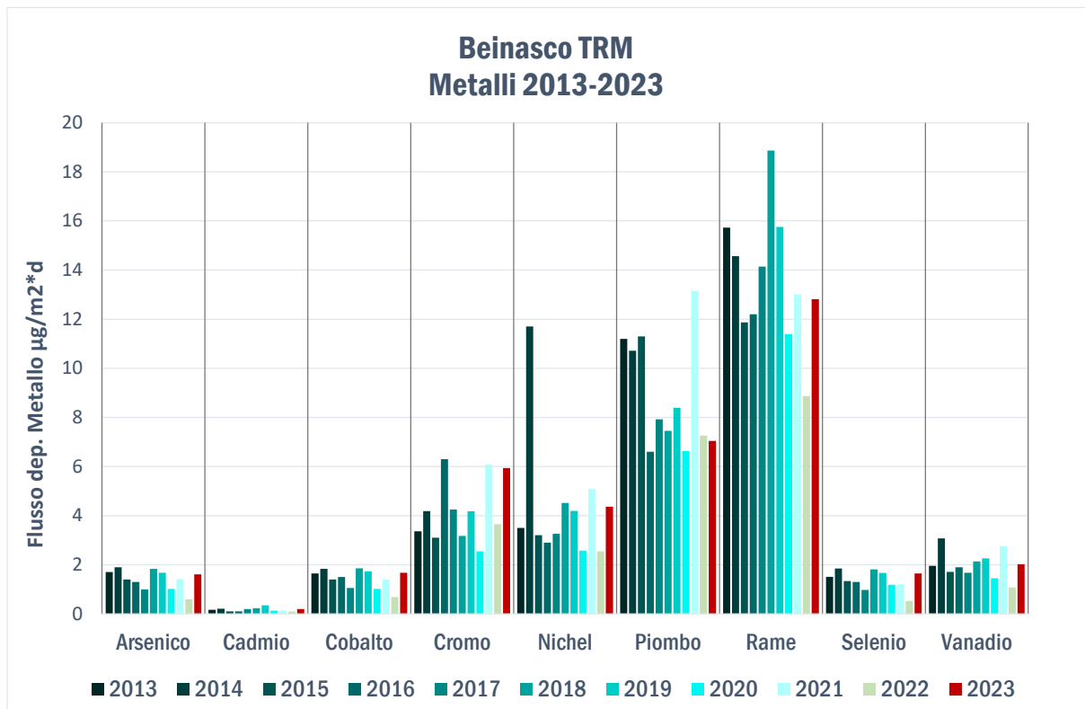
Figura 39 - Deposizioni metalli 2013-2023 nel sito di Beinasco Aldo Mei
