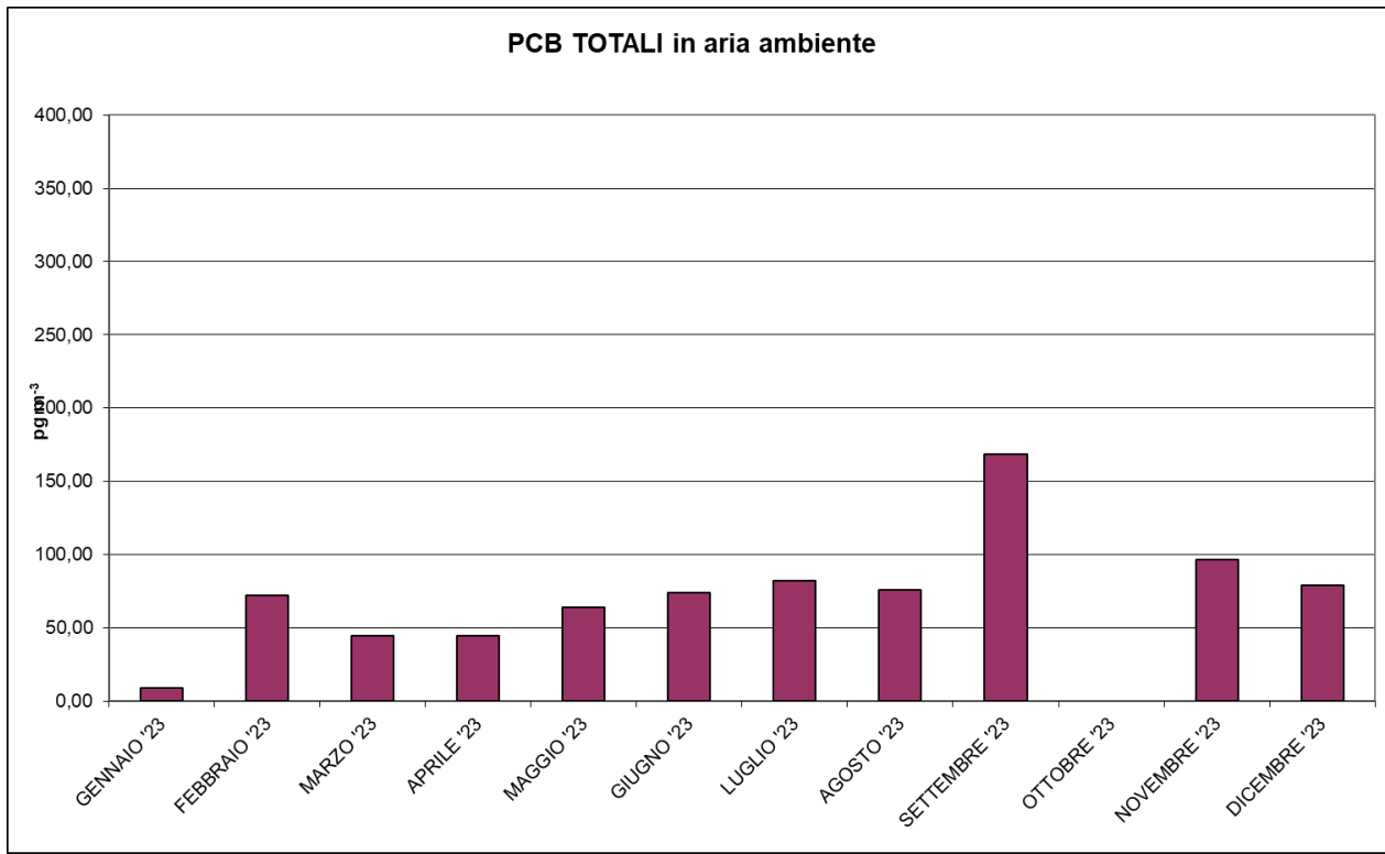
Figura 25 - Concentrazioni di PCB Totali in aria ambiente anno 2023
