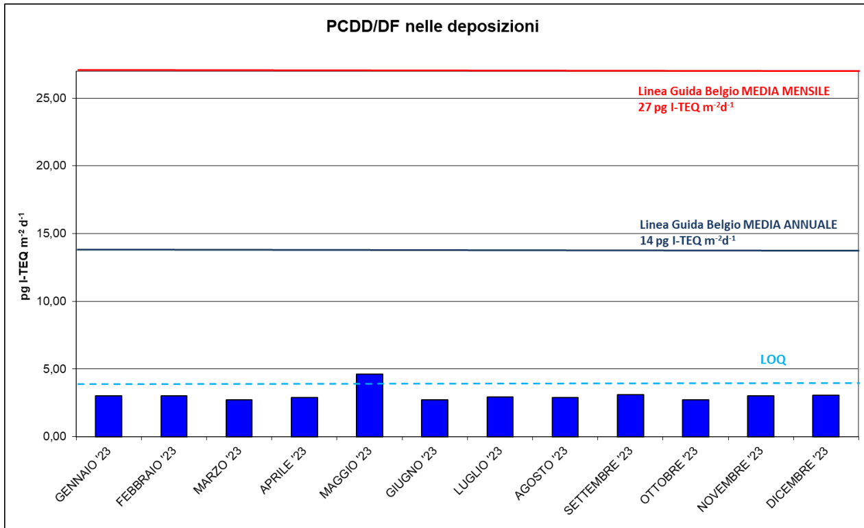
Figura 45 - Concentrazioni di PCDD e PCDF nelle deposizioni mensili anno 2023
