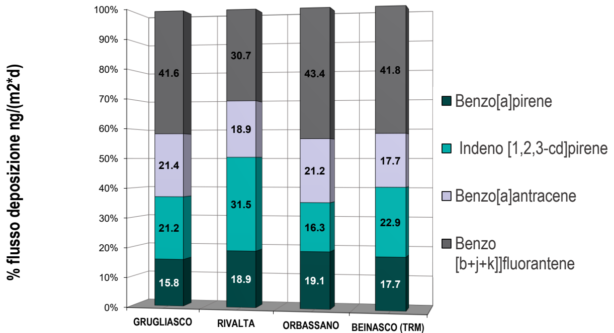
Figura 31 - Grafico di confronto ratei flussi deposizioni nel 2023
