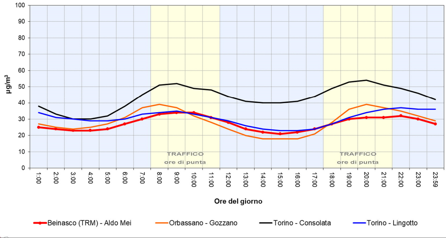
NO2: Andamento del giorno medio - anno 2021 confronto cabina TRM e stazioni della Rete Regionale di Rilevamento della Qualità dell'Aria
