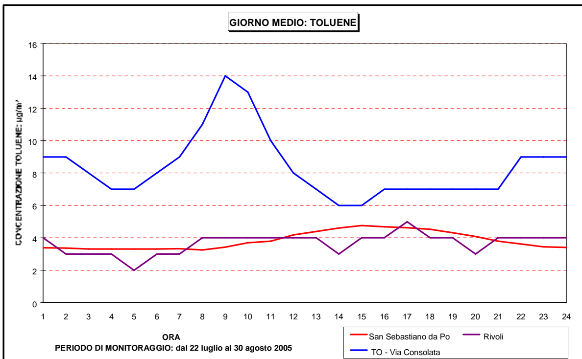
Figura 27: Toluene andamento giorno medio confronto con i dati delle stazioni di Torino via della Consolata e Rivoli
