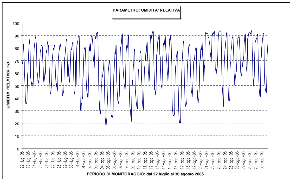
Figura 7: Umidità Relativa
