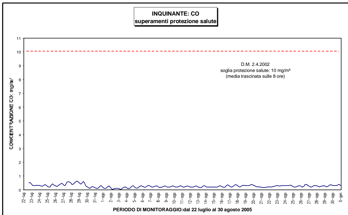
Figura 21: CO Confronto con il limite di legge (media trascinata su 8 ore)
