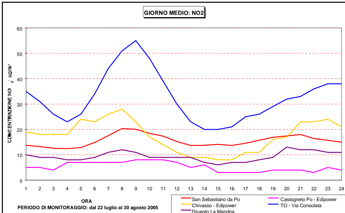
Figura 16: NO andamento orario, confronto con i dati delle centraline di Torino-via della Consolata, Edipower Chivasso e Edipower Castagneto Po.
