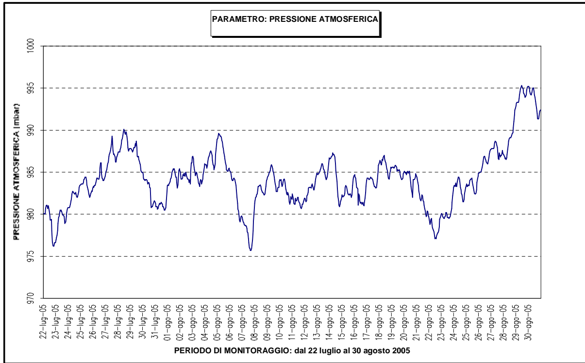
Figura 6: Pressione Atmosferica
