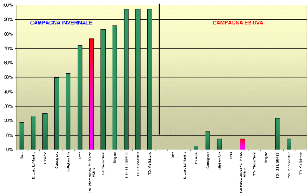
Figura 42: Percentuali di superamento del limite giornaliero per la protezione della salute nella provincia di Torino (periodi: 8/12/04 – 12/01/05 e 22/07/05 – 30/08/05)
