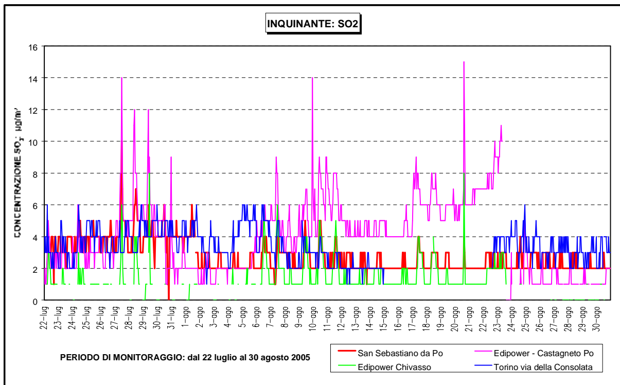
Figura 12: SO 2 andamento medie orarie e confronto con i dati della stazione di Torino in via Consolata e le centraline Edipower di Castagneto Po e di Chivasso.
