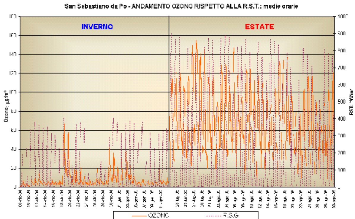
Figura 38: Andamento orario dell'ozono rispetto alla radiazione solare totale nelle due campagne di monitoraggio
