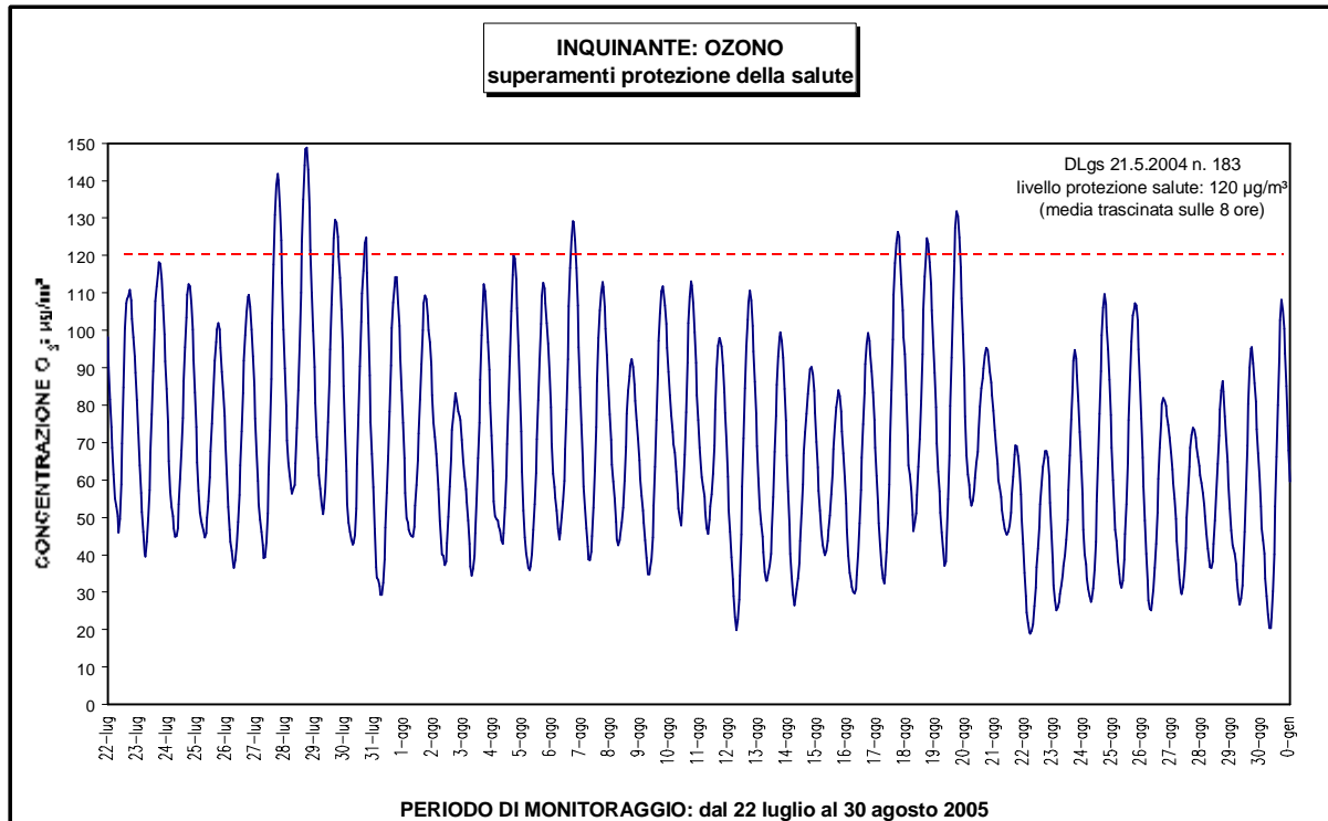
Figura 20: O 3 confronto con il livello di protezione salute umana (media trascinata sulle 8 ore)
