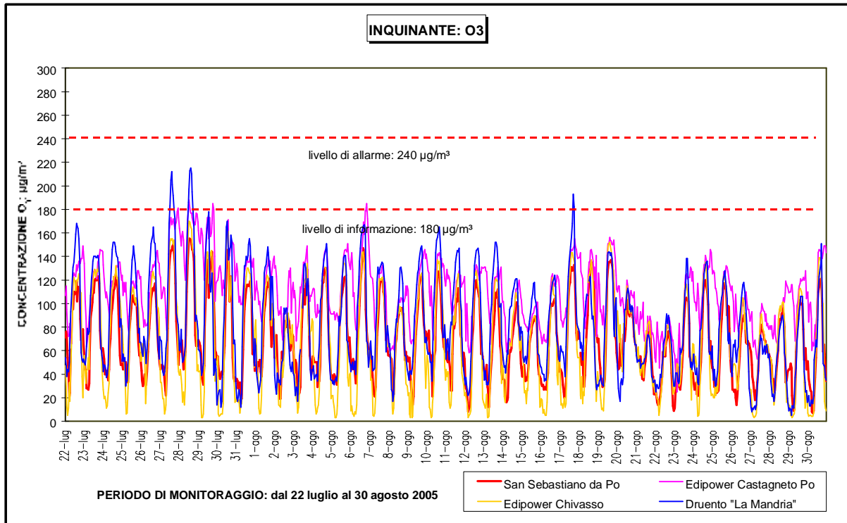
Figura 18: O 3 (medie orarie) confronto con i limiti di legge, livello di informazione, livello di allarme e con i dati delle centraline di Druento "La Mandria", Edipower Chivasso e Edipower Castagneto Po.
