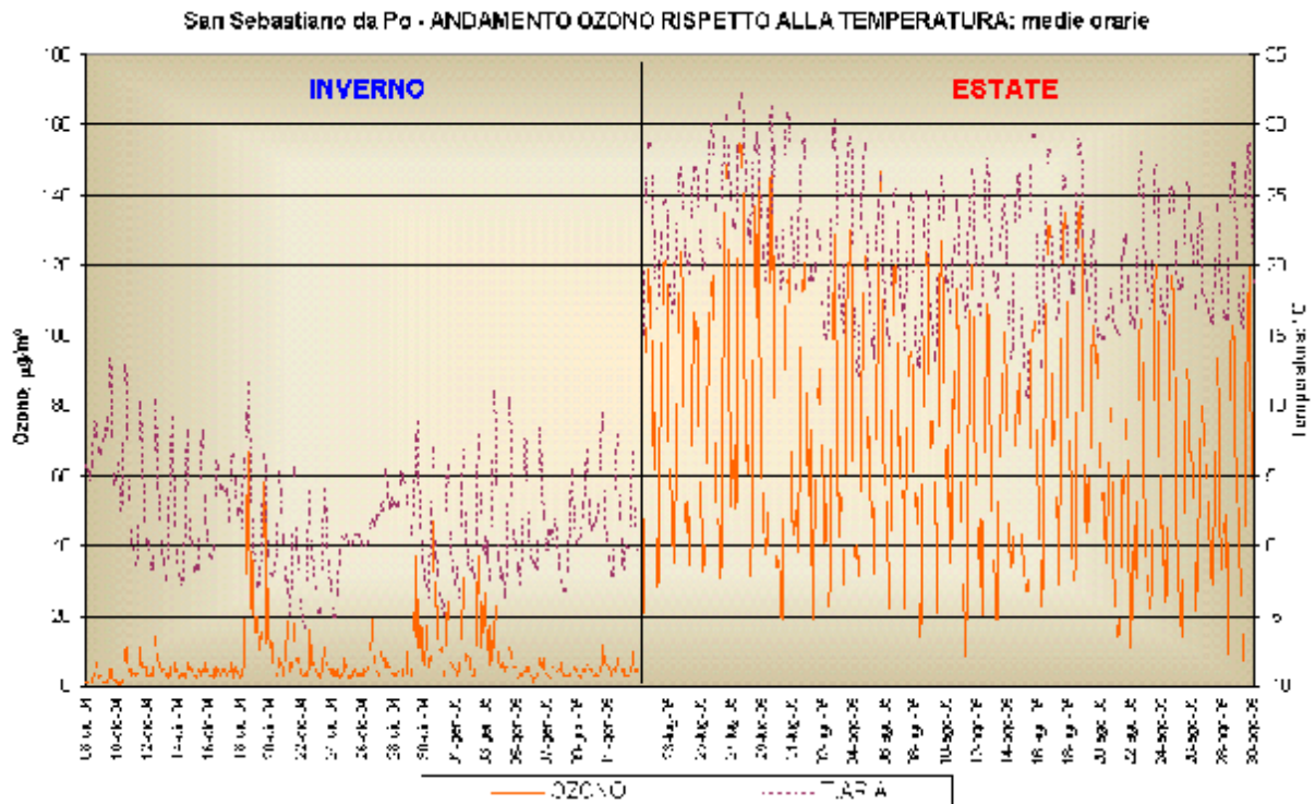
Figura 37: Andamento orario dell'ozono rispetto alla temperatura dell'aria nelle due campagne di monitoraggio
