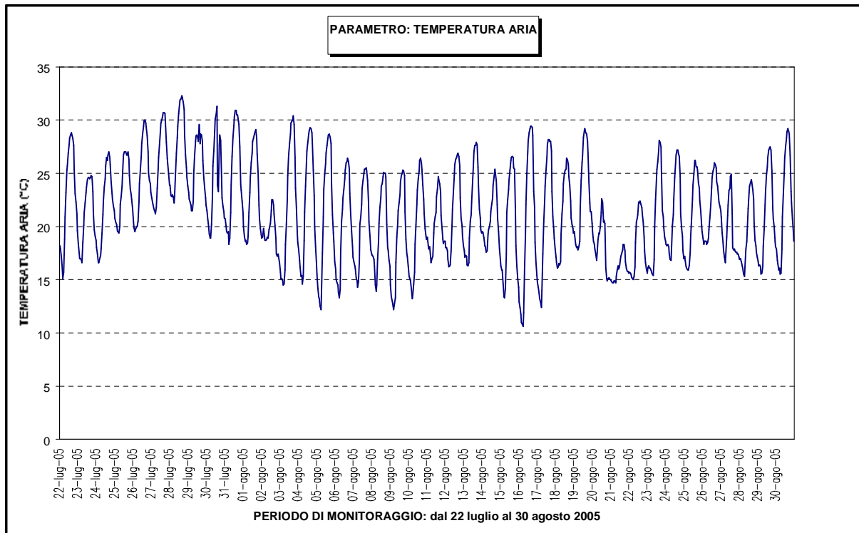
Figura 8: Temperatura aria
