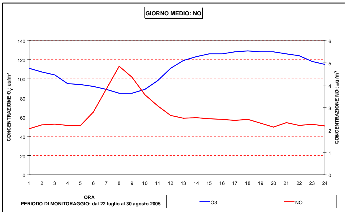
Figura 19: O 3 NO Andamento giorno medio
