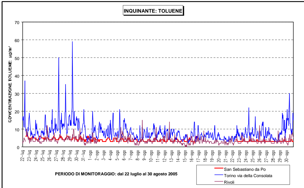
Figura 26: Toluene andamento orario, confronto con i dati delle stazioni di Torino via della Consolata e Rivoli
