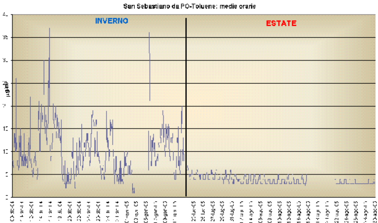
Figura 33: Medie orarie di Toluene rilevate nelle due campagne di monitoraggio
