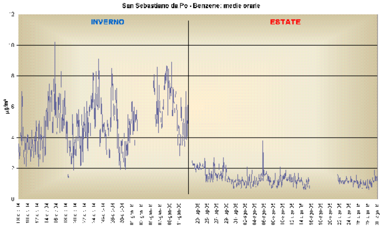
Figura 32 : Medie orarie di Benzene rilevate nelle due campagne di monitoraggio
