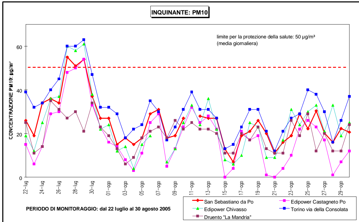
Figura 28: PM10 andamento giornaliero, confronto con limite di legge e con alcune stazioni fisse della rete di monitoraggio
