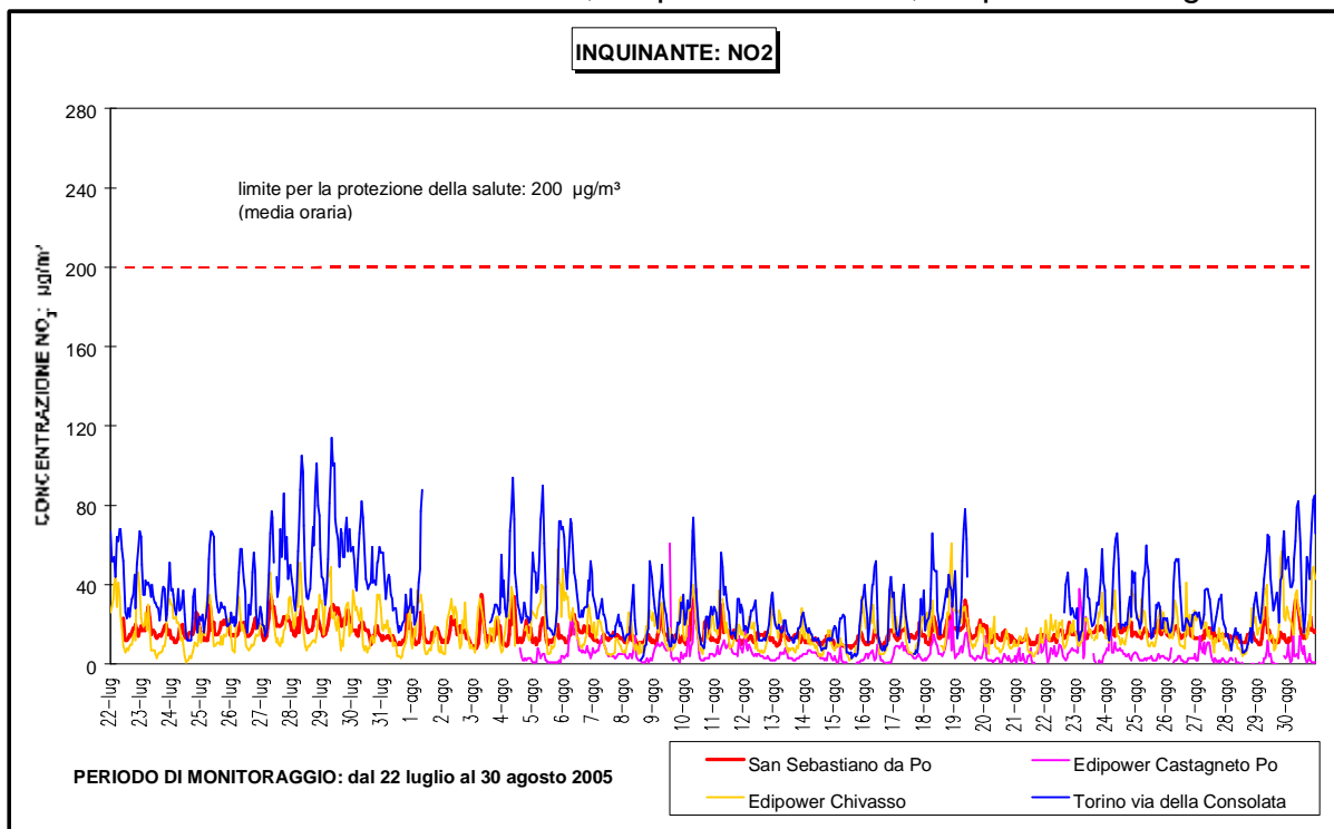
Figura 14: NO 2 andamento orario confronto con i limiti di legge e i dati della stazione di Torino-via della Consolata, Edipower Chivasso, Edipower Castagneto Po.
