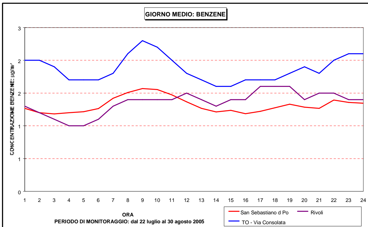
Figura 25 : Benzene andamento giorno medio confronto con i dati di Torino via della Consolata e Rivoli
