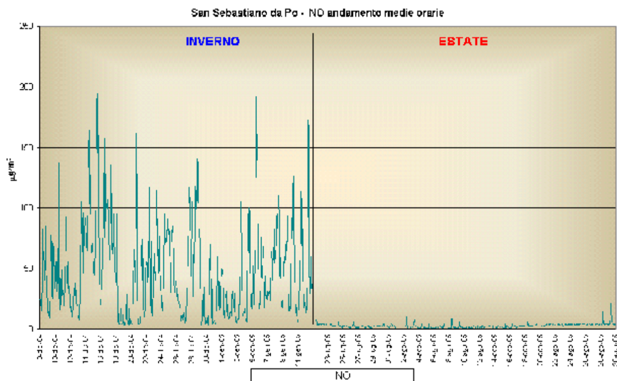
Figura 34: Medie orarie di NO rilevate nelle due campagne di monitoraggio
