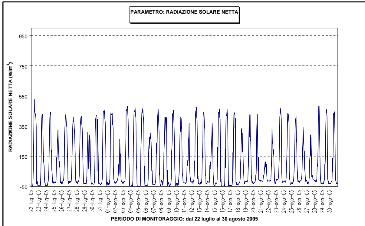
Figura 10: Radiazione Solare Netta
