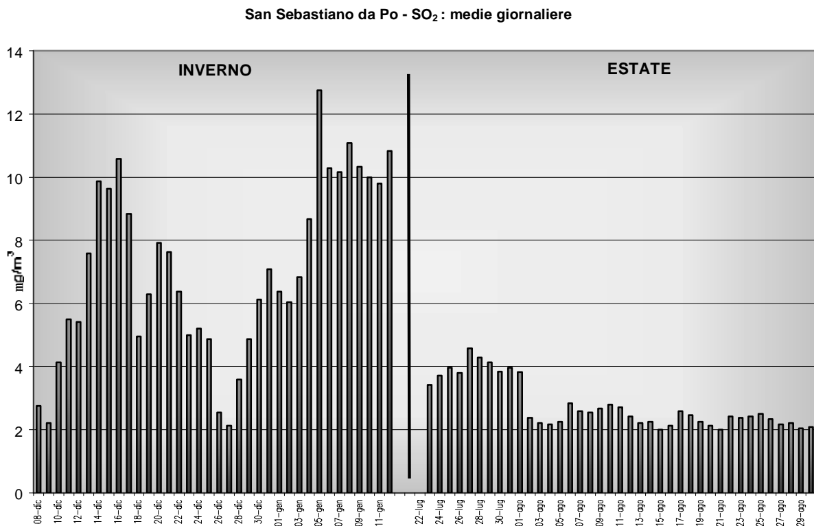
Figura 30: Medie giornaliere di SO 2 rilevate nelle due campagne di monitoraggio
