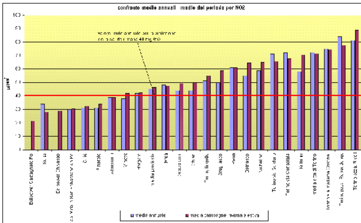
Figura 36: Concentrazioni medie annuali e media periodo (08/12/04 - 12/01/05) e (22/07/05 - 30/08/05) di NO 2 nella provincia di Torino. (Per San Sebastiano da Po: media annuale stimata come in Nota 1)
