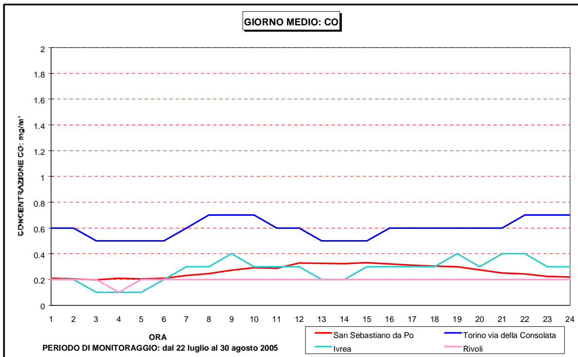
Figura 23: CO andamento giorno medio
