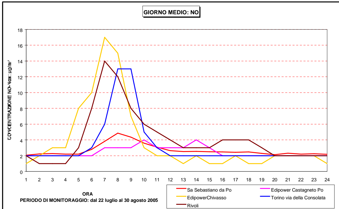
Figura 17: NO andamento giorno medio, confronto con i dati registrati in Torino-via della Consolata, Rivoli e le centraline Edipower di Castagneto Po e Chivasso
