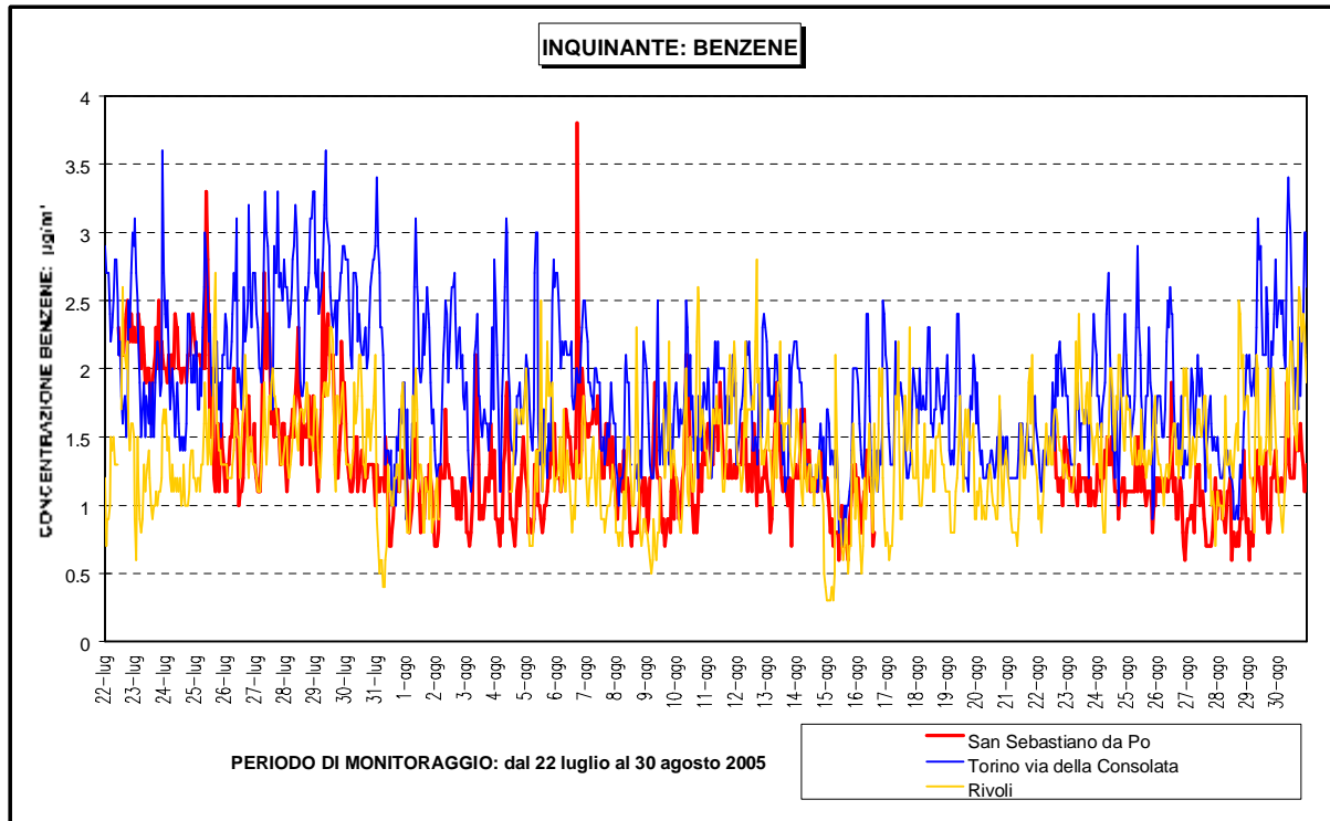
Figura 24 :Benzene andamento orario, confronto con i dati delle stazioni di Torino-via della Consolata e Rivoli
