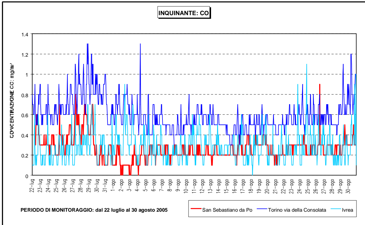
Figura 22: CO andamento orario, confronto con i dati delle stazioni di Torino-via della Consolata e Ivrea
