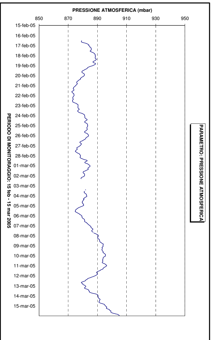
Figura 6: Pressione Atmosferica
