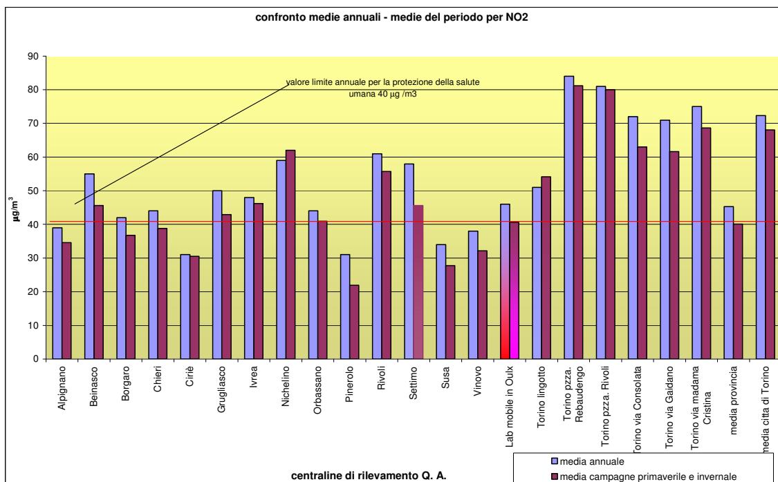
Figura 33: Concentrazioni medie annuali e media del periodo delle due campagne di rilevamento per NO 2 nella provincia di Torino. (Per Oulx: media annuale stimata come in Nota 1)
