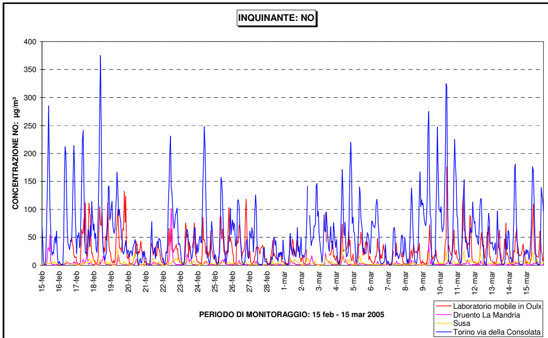
Figura 15: NO andamento orario, confronto con i dati delle centralina di Torino via della Consolata, Susa e Druento La Mandria.
