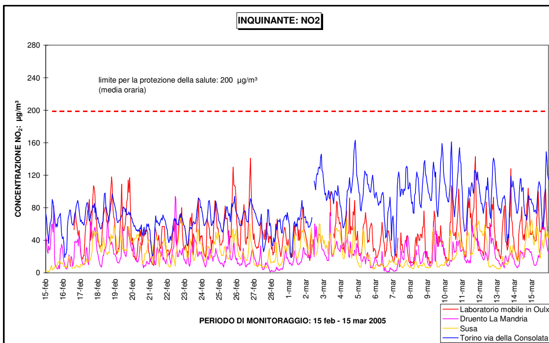
Figura 13: NO 2 andamento orario, confronto con i dati di alcune delle stazioni della rete fissa di rilevamento della qualità dell'aria regionale e dei limiti di legge
