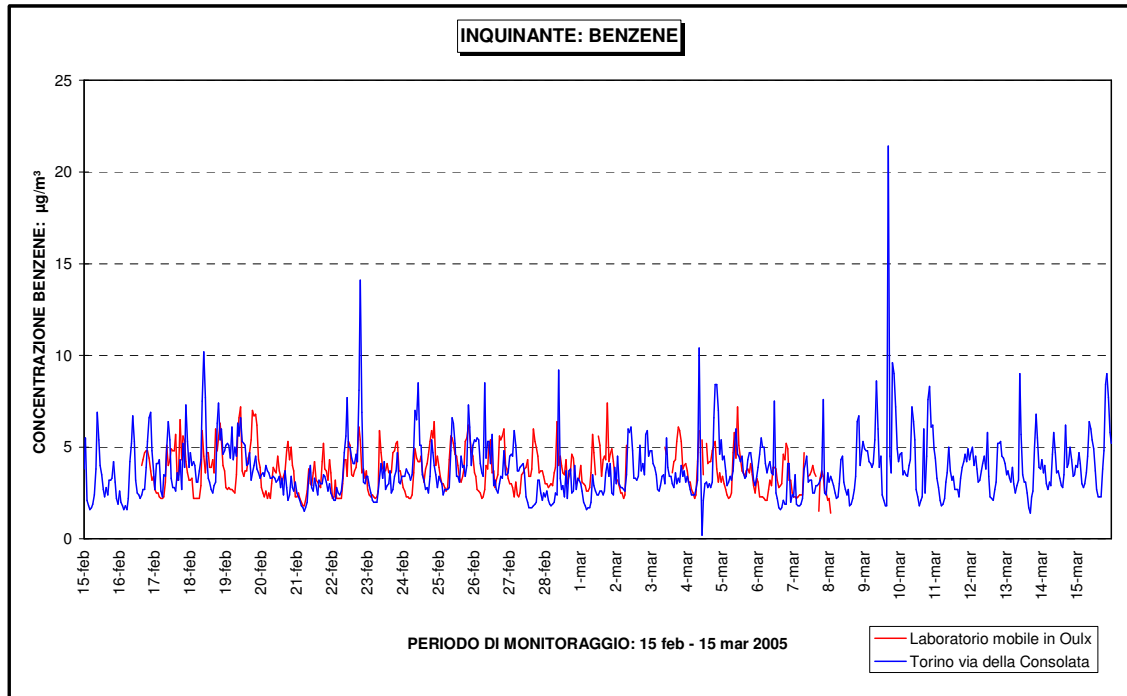
Figura 23 :Benzene andamento orario, confronto con i dati della stazione di Torino via della Consolata.
