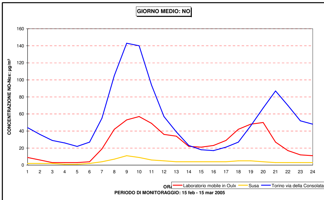
Figura 16: NO andamento giorno medio confronto con i dati delle centralina di Torino via della Consolata, e Susa.
