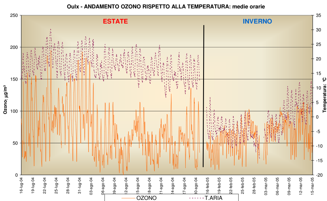
Figura 34: Andamento orario dell'ozono rispetto alla temperatura dell'aria nelle due campagne di monitoraggio
