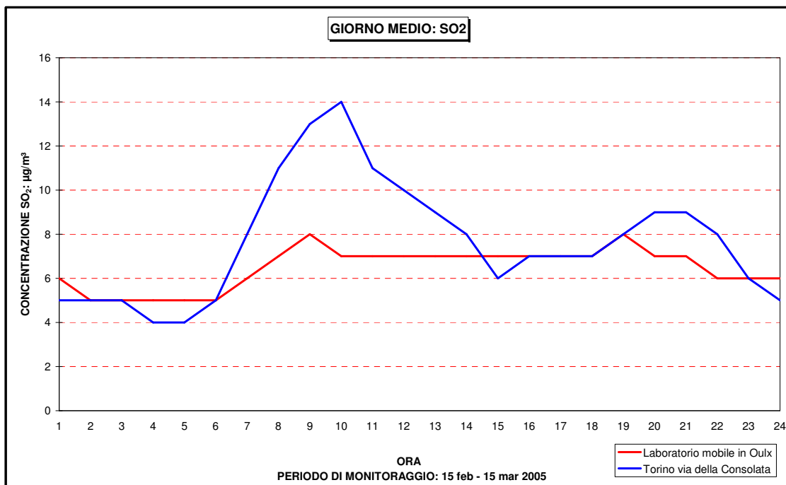
Figura 12: SO 2 andamento giorno medio confronto con i dati della stazione di Torino via della Consolata
