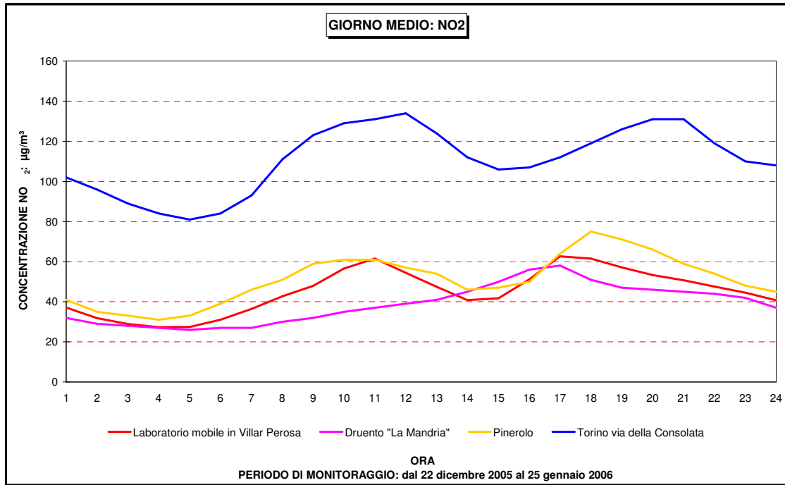
Figura 24: NO 2 andamento giorno medio campagna invernale.
