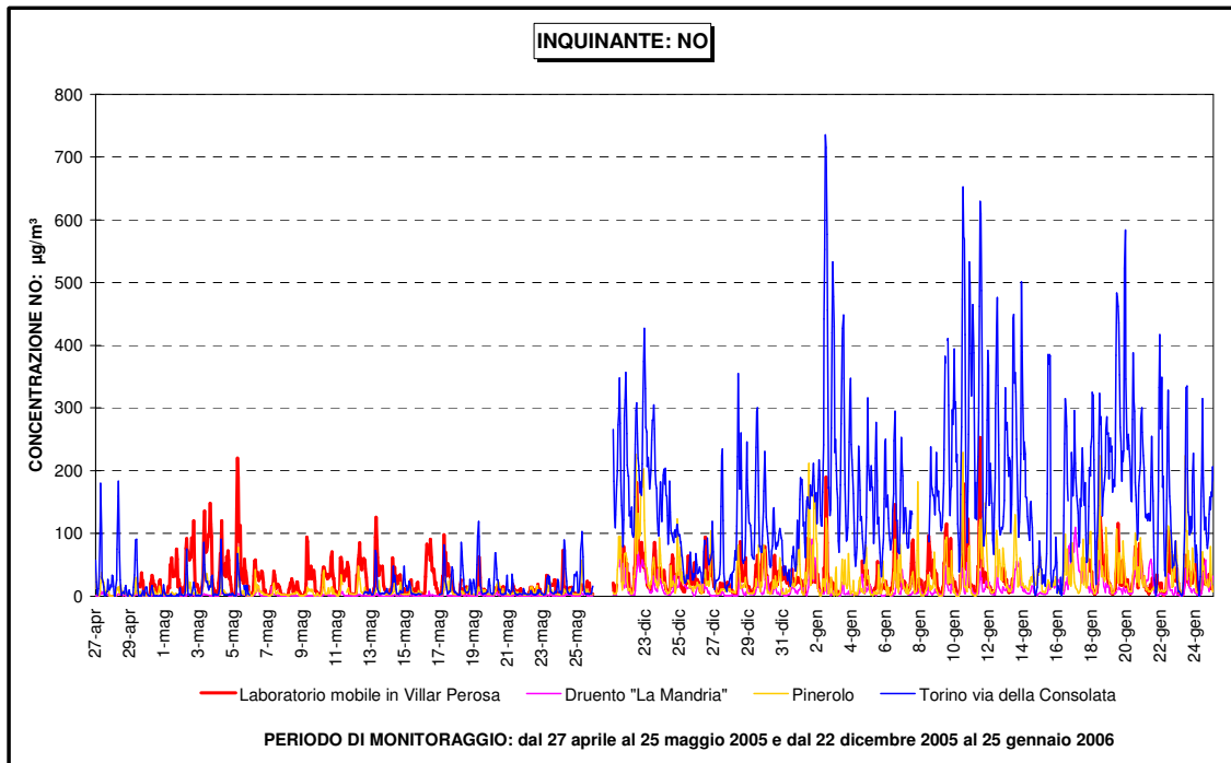
Figura 25: NO andamento orario, confronto con i dati delle centraline di Torino-via della Consolata, Druento "La Mandria" e Pinerolo.
