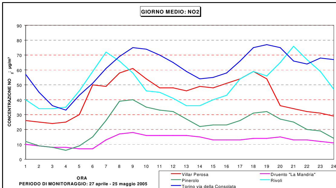
Figura 23: NO 2 andamento giorno medio campagna primaverile, confronto con i dati i alcune stazioni di rilevamento della qualità dell'aria.
