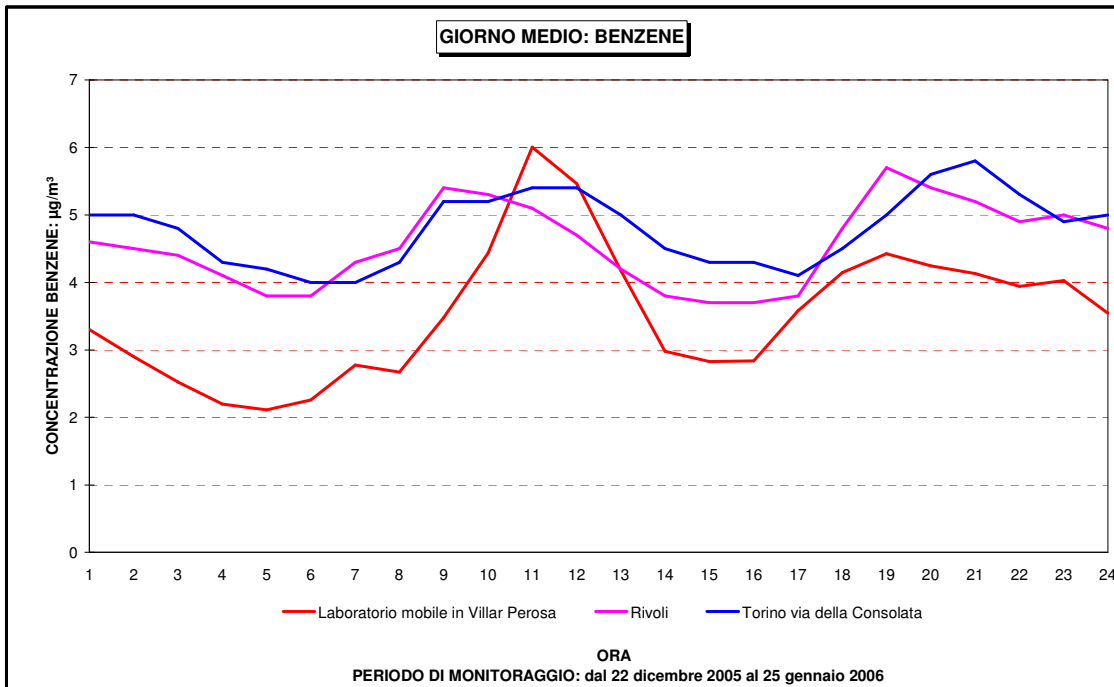
Figura 40: Benzene andamento giorno medio periodo invernale confronto con i dati di Torino via della Consolata e Rivoli
