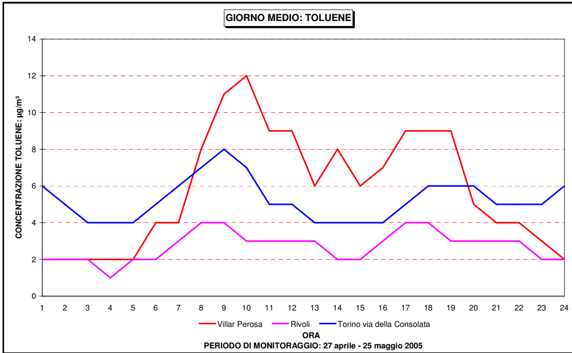
Figura 41: Toluene andamento giorno medio campagna primaverile confronto con i dati delle stazioni di Torino via della Consolata e Rivoli
