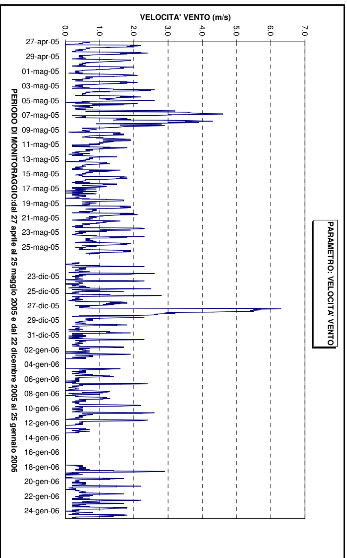
Figura 8: Parametro Velocità Vento
