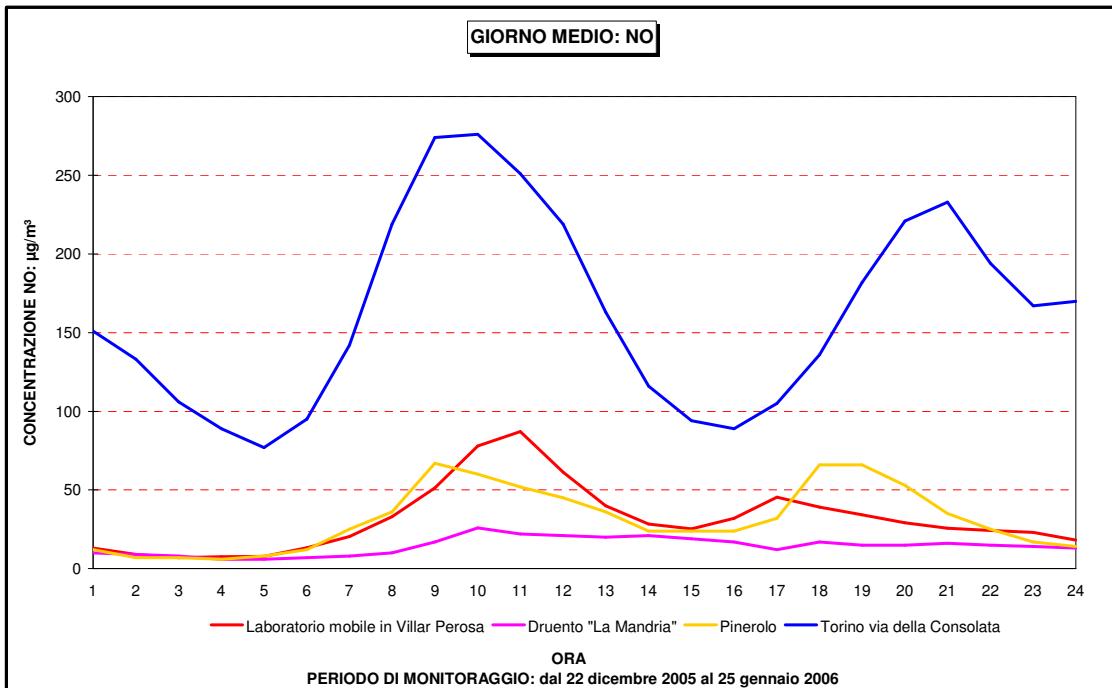
Figura 27: NO giorno medio campagna invernale
