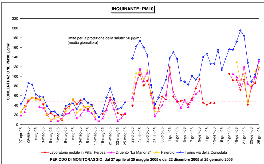
Figura 43: Medie giornaliere di PM10 rilevate nelle due campagne di monitoraggio
