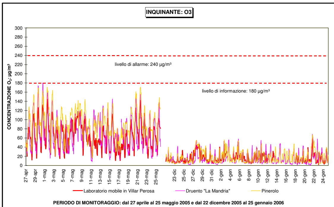
Figura 35: O 3 (medie orarie) confronto con i limiti di legge, livello di informazione, livello di allarme e con i dati della centralina di Pinerolo e Druento “La Mandria”
