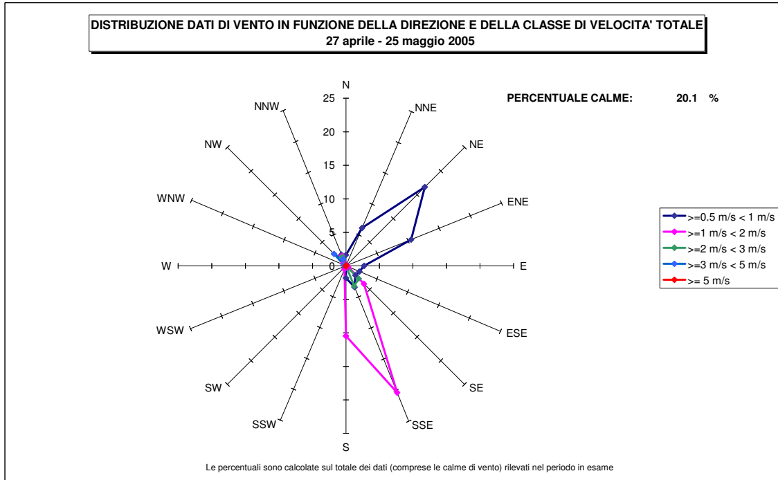
Figura 2: Distribuzione dati di vento in funzione della direzione e della classe di velocità totale I campagna
