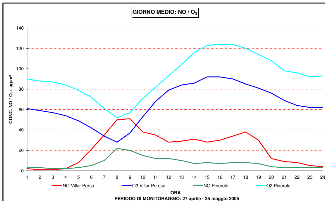
Figura 29: NO x / O 3 confronto giorno medio periodo primaverile
