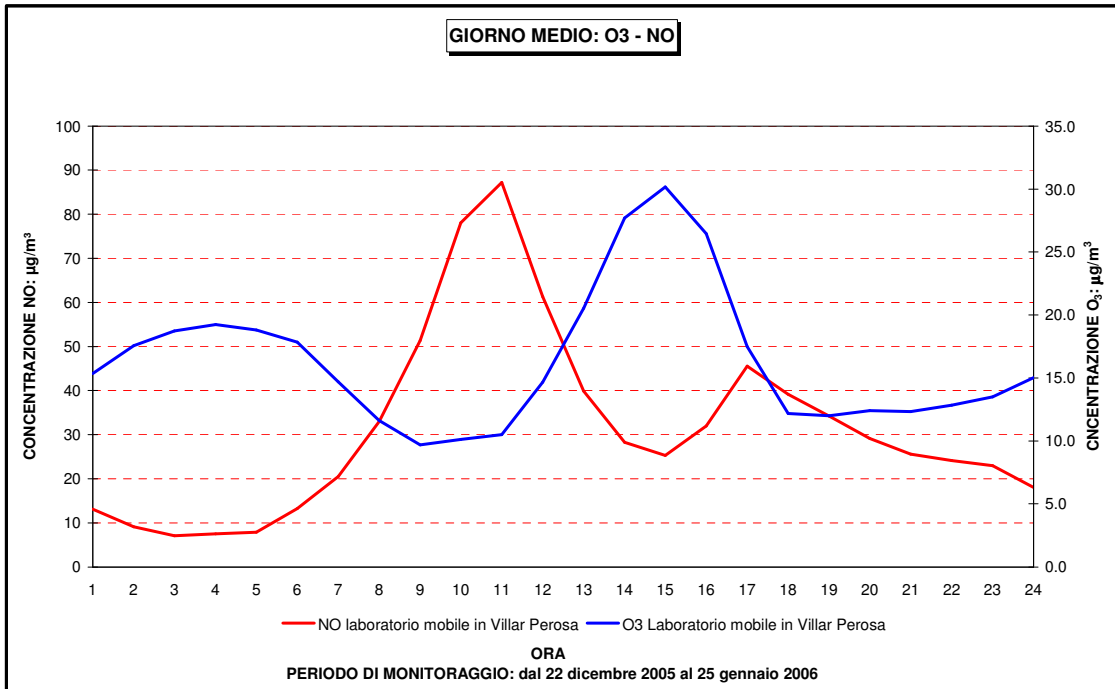
Figura 30: NO O 3 confronto giorno medio periodo invernale
