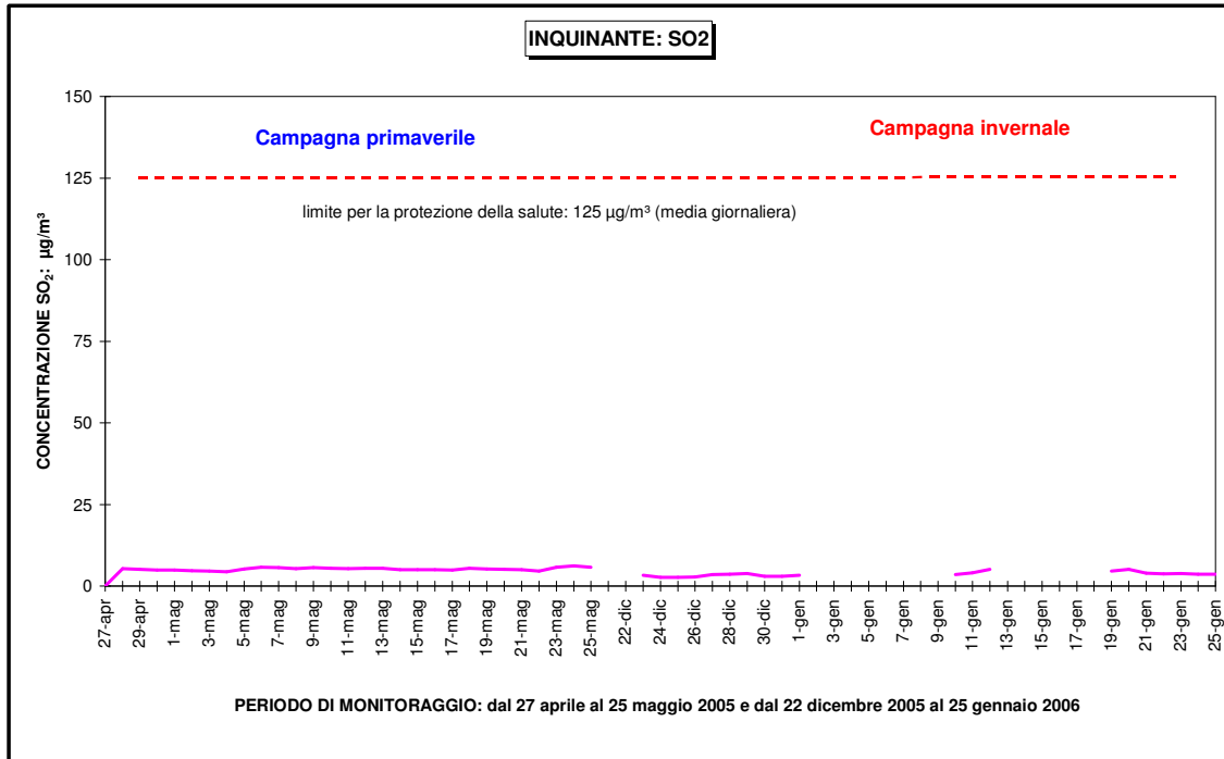
Figura 16: SO 2 andamento medie orarie e confronto con i dati della centralina di rilevamento della qualità dell'aria di Torino in via della Consolata.
