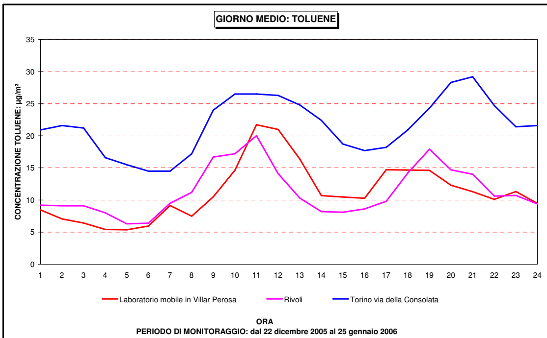
Figura 42: Toluene andamento giorno medio campagna invernale confronto con i dati delle stazioni di Torino via della Consolata e Rivoli
