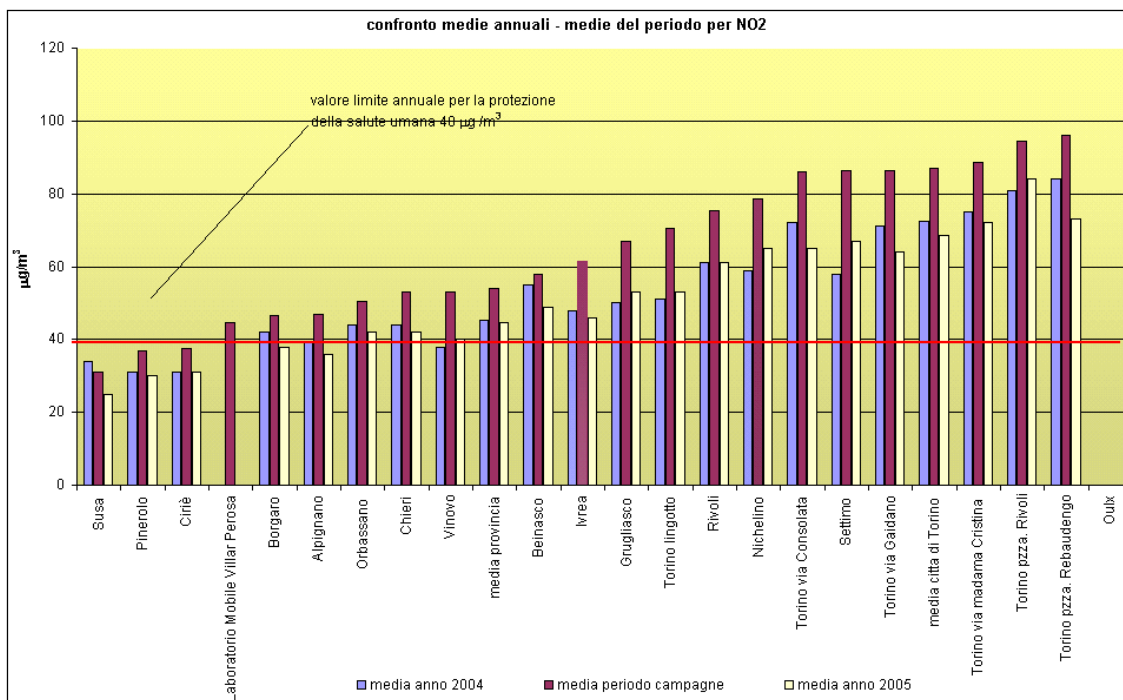
Figura 28: Concentrazioni medie annuali e media periodo (27/04/2005 - 25/05/2005) e (22/12/2005 - 25/01/2006) di NO 2 nella provincia di Torino.
