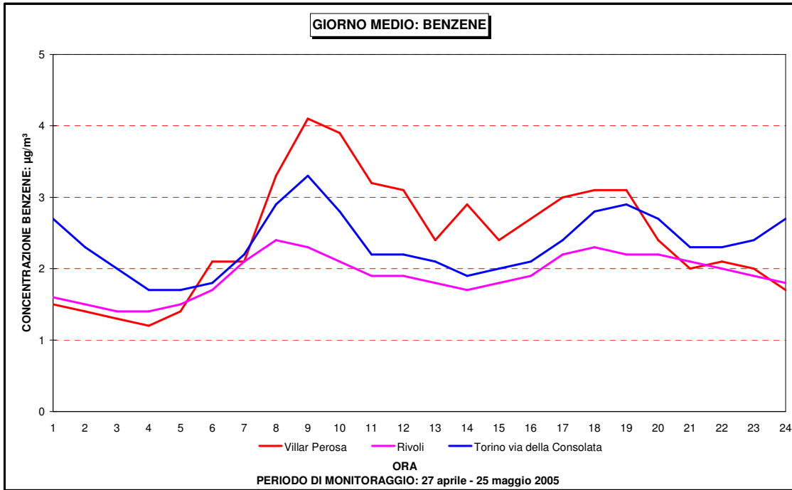
Figura 39: Benzene andamento giorno medio campagna primaverile confronto con i dati di Torino via della Consolata e Rivoli
