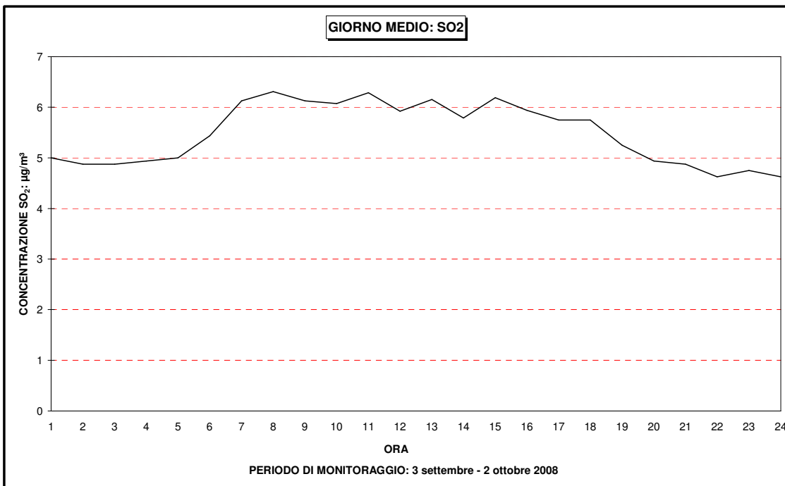
Figura 13 – SO 2 : andamento del giorno medio
