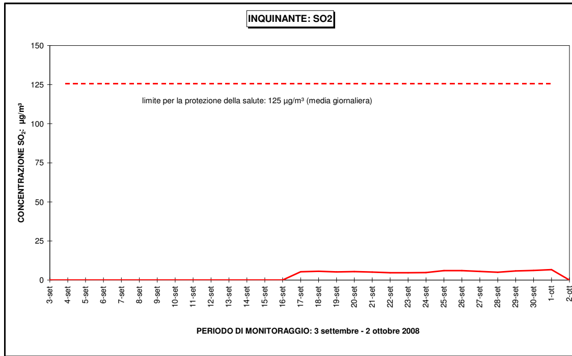
Figura 12 – SO 2 : andamento orario
