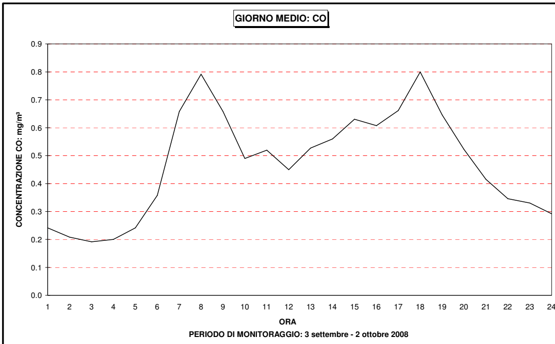
Figura 15 – CO: andamento del giorno medio
