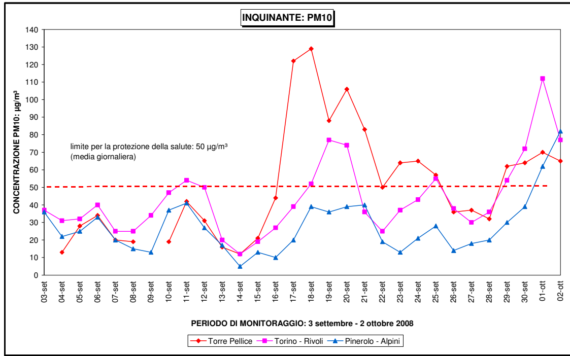
Figura 23– Particolato sospeso PM 10 : confronto con il limite giornaliero per la protezione della salute e con i dati delle stazioni di Torino-Rivoli e Pinerolo.
