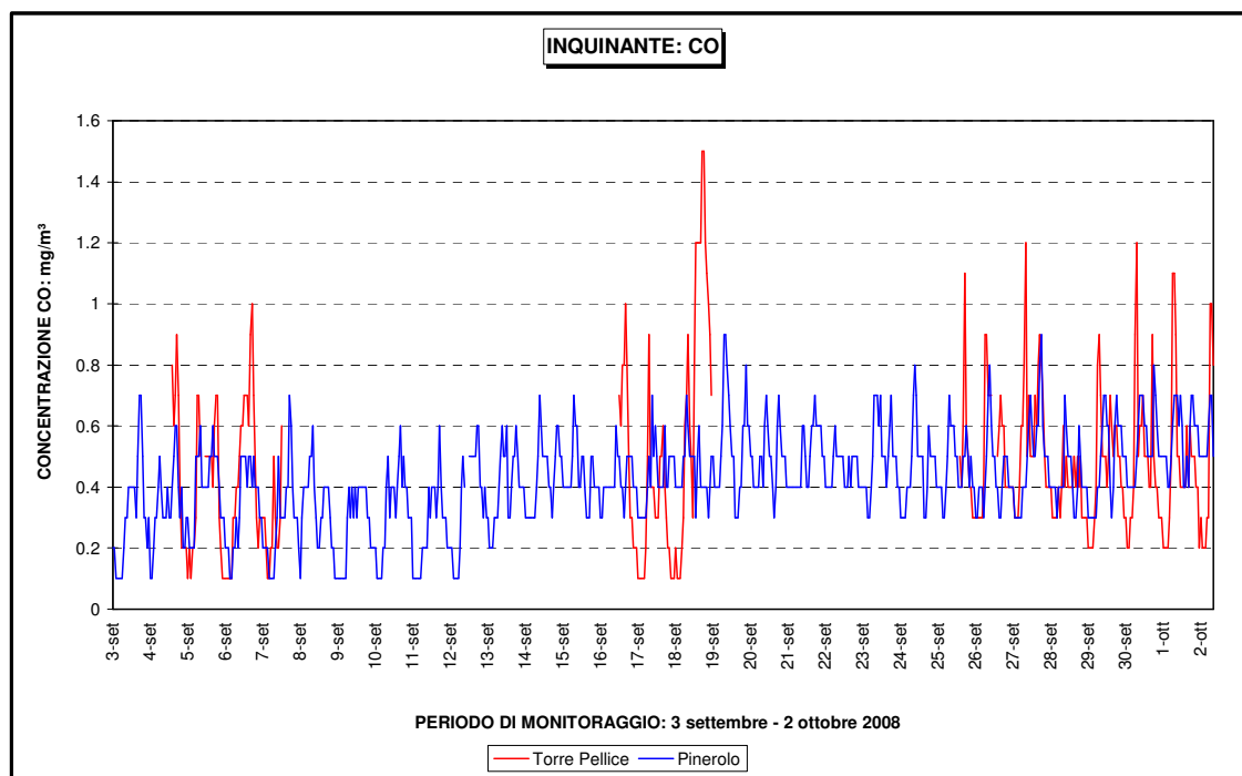
Figura 14– CO: andamento orario, confronto con la stazione di Pinerolo.
