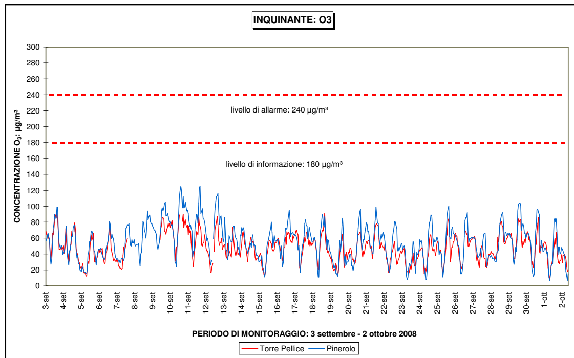
Figura 24– O 3 : confronto con i limiti di legge e con la stazione di Pinerolo
