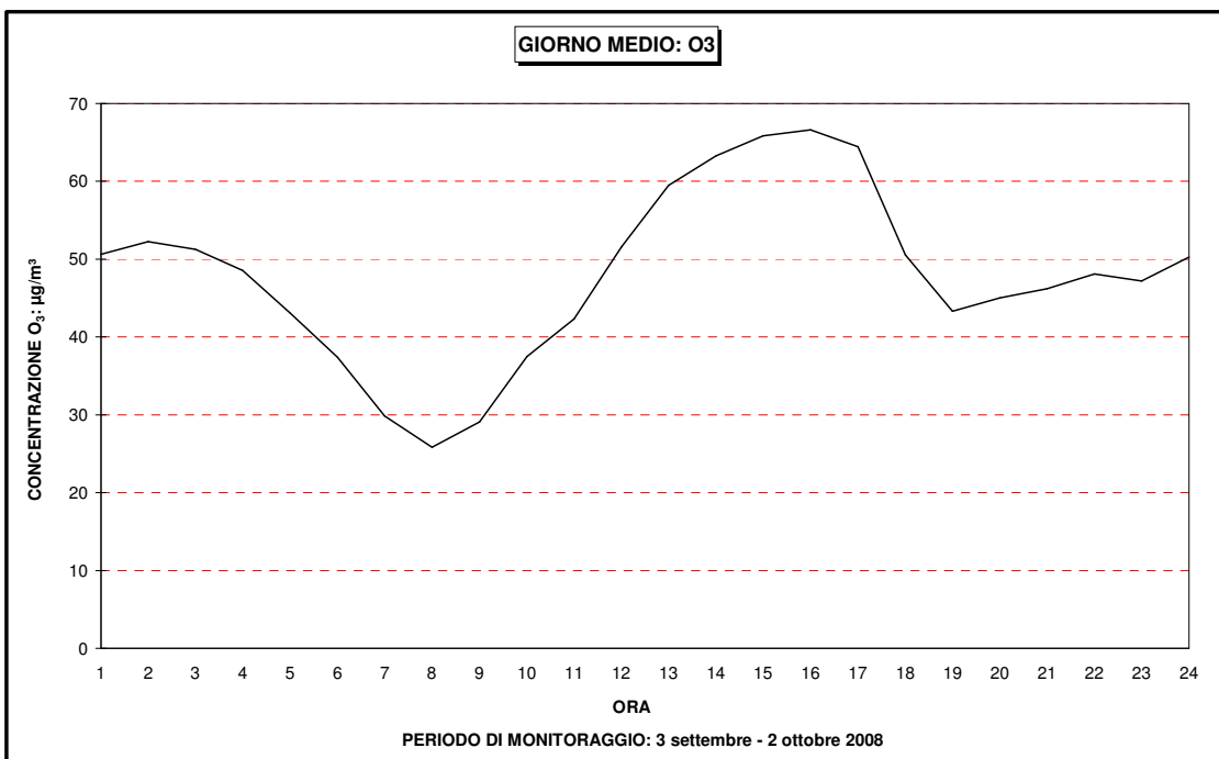
Figura 25– O 3 : andamento del giorno medio
