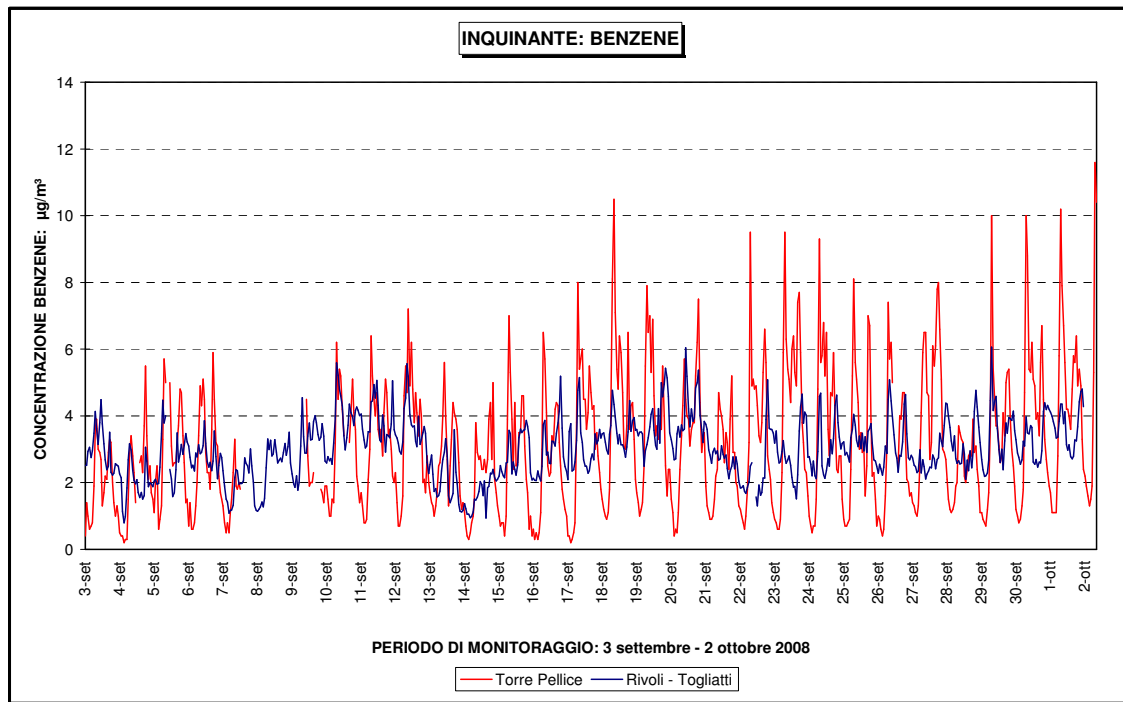
Figura 20– Benzene: andamento della concentrazione oraria e confronto con i dati di Rivoli.
