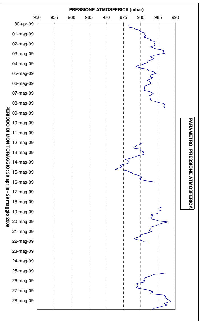
Figura 6: Pressione Atmosferica
