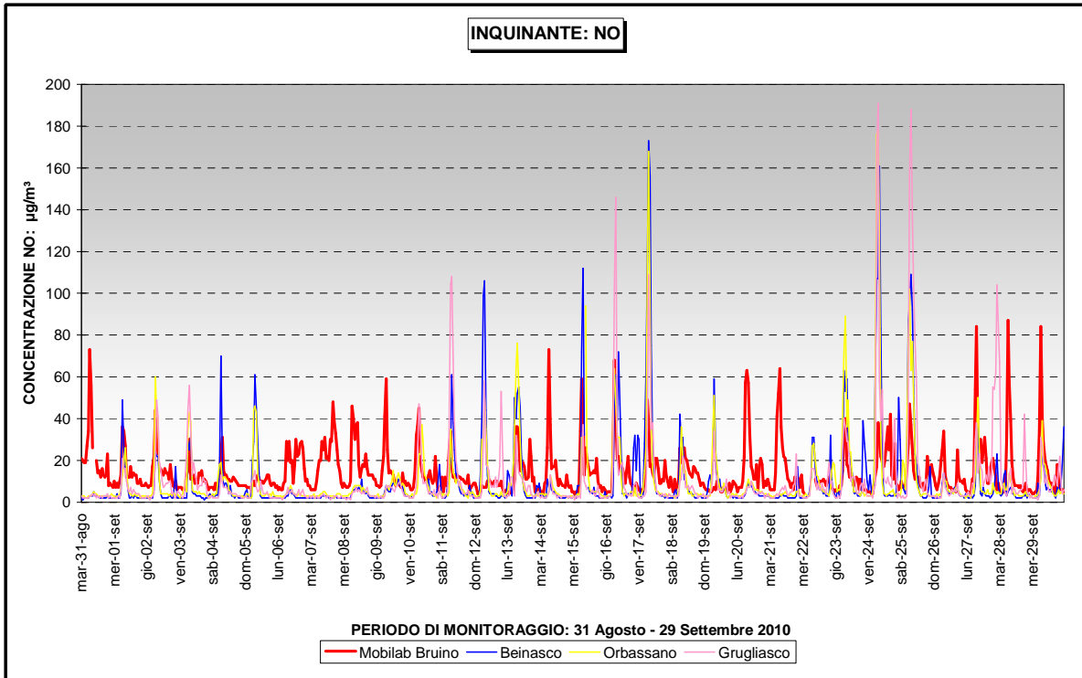
Figura 14– NO: andamento della concentrazione oraria
