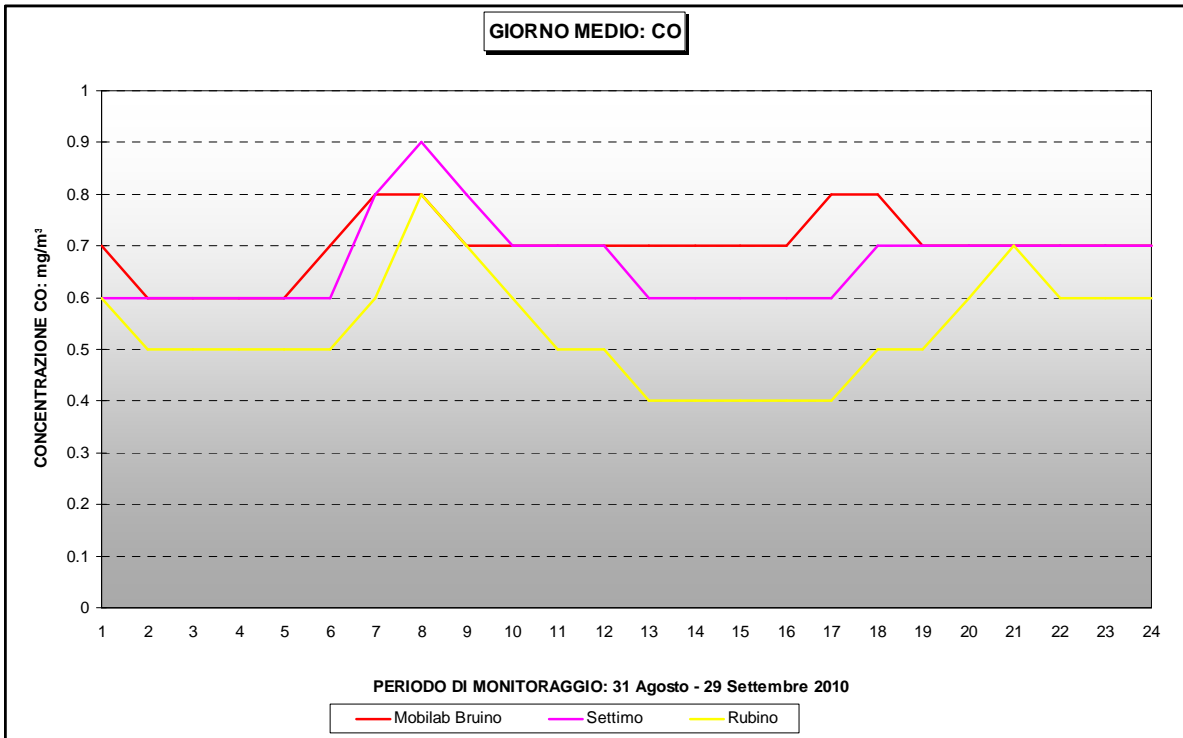
Figura 13 – CO: andamento del giorno medio
