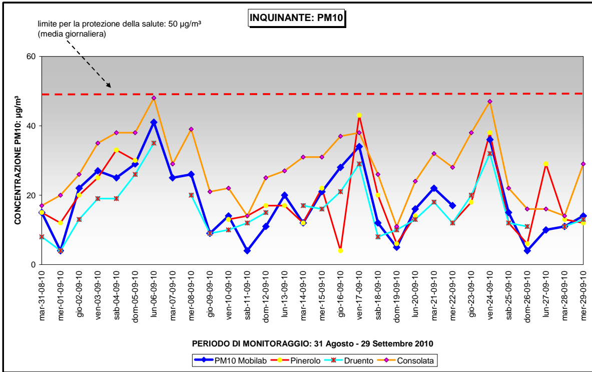
Figura 18– Particolato sospeso PM 10 : confronto con il limite giornaliero per la protezione della salute e con i dati delle stazioni di Pinerolo, Druento e Torino Consolata.
