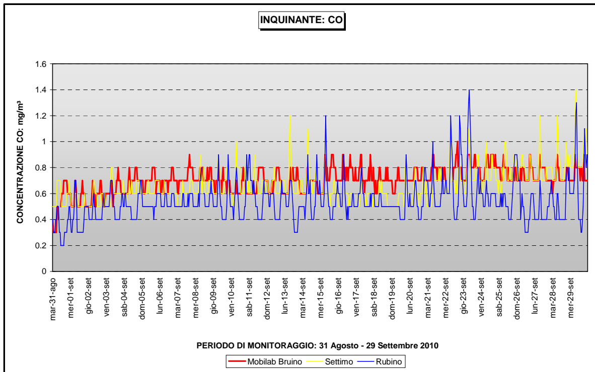
Figura 12– CO: andamento orario.
