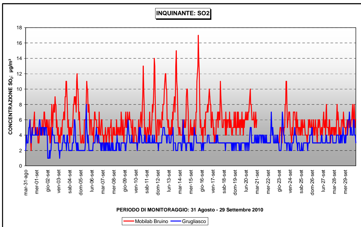
Figura 10 – SO 2 : andamento orario
