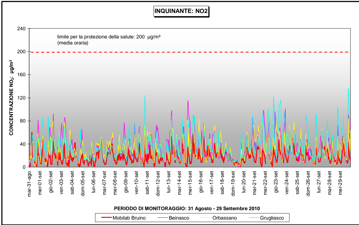
Figura 16– NO 2 : confronto con i limiti di legge
