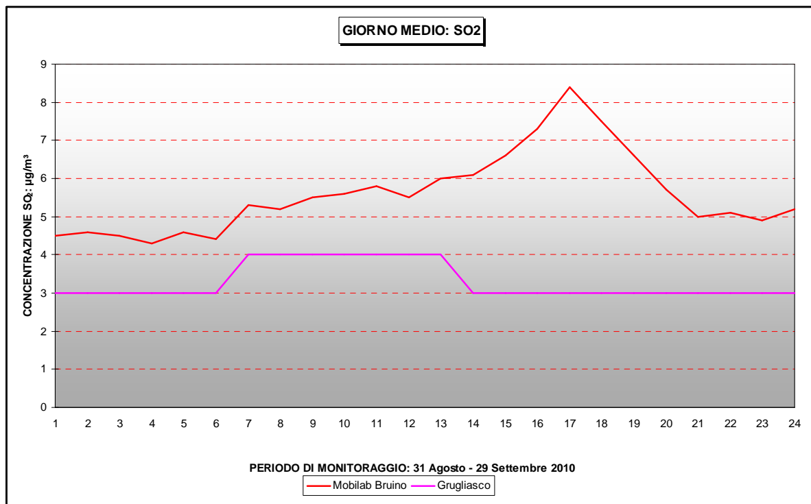
Figura 11 – SO 2 : andamento del giorno medio
