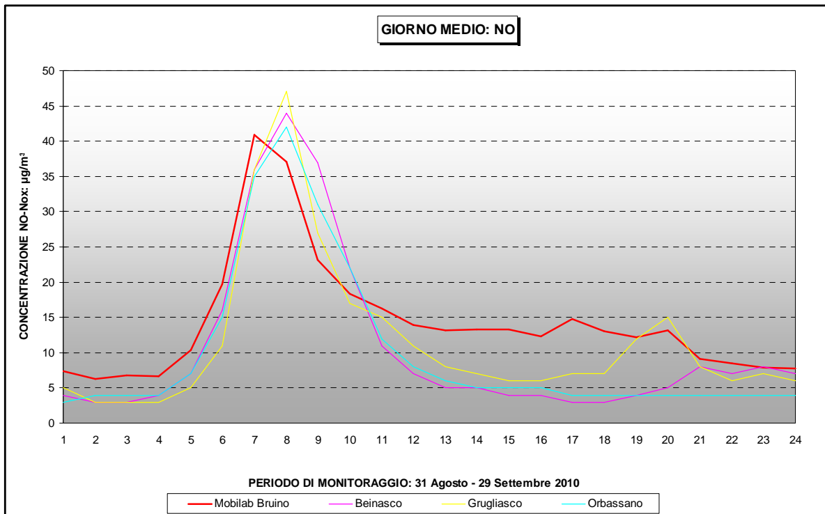
Figura 15– NO: andamento del giorno medio
