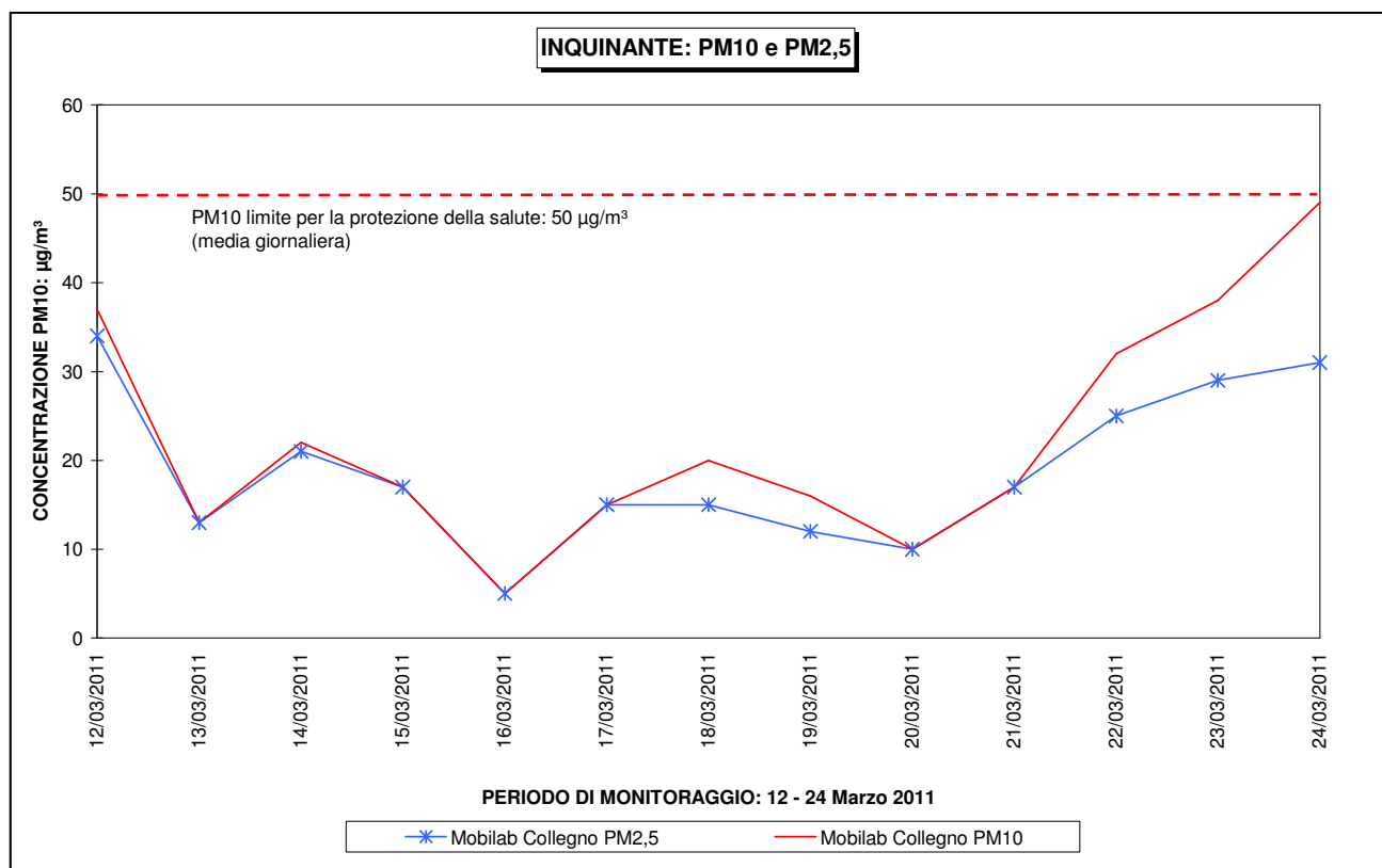
Figura 21 – Particolato sospeso \text{PM}_{10} e \text{PM}_{2,5} : confronto con il limite giornaliero per la protezione della salute
