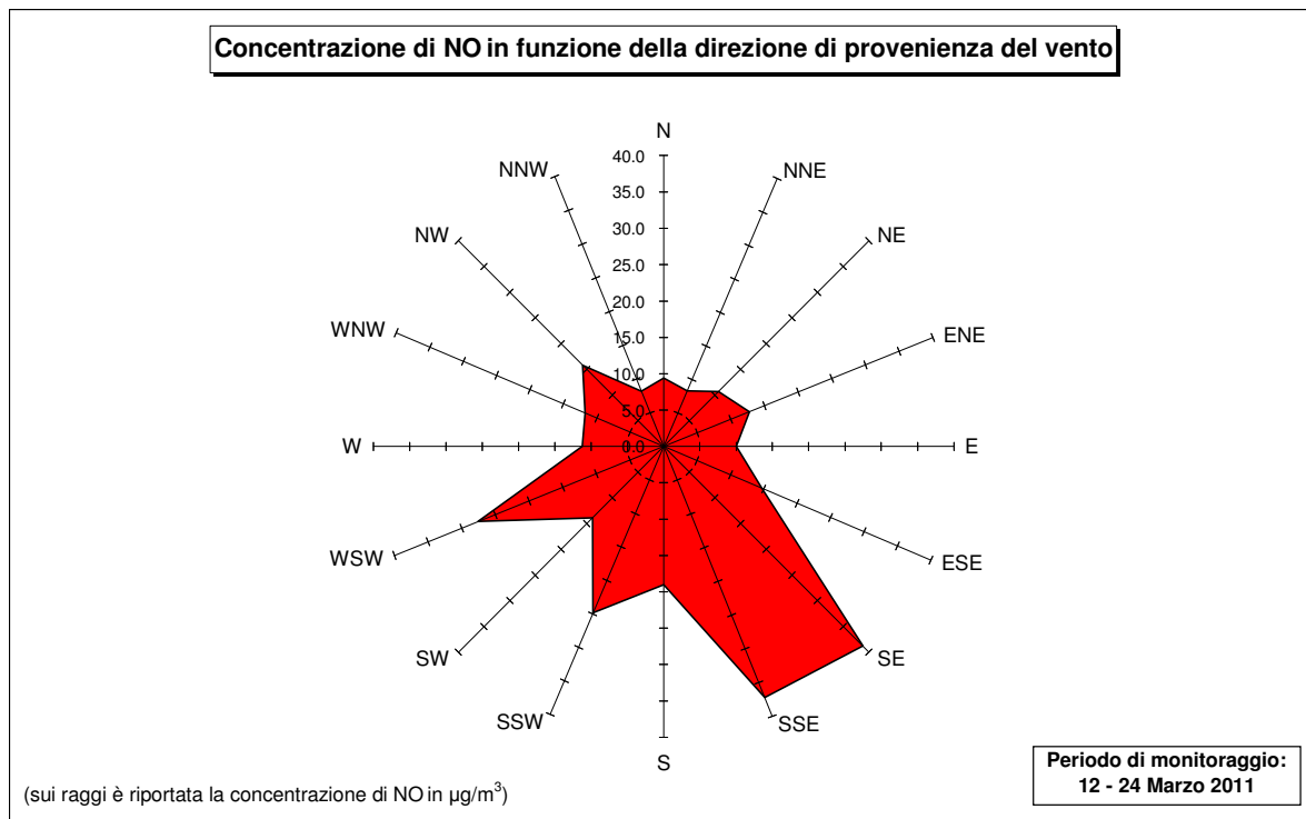
Figura 27 – Concentrazioni di NO in funzione della direzione di provenienza del vento nel corso della campagna di monitoraggio nel Comune di Collegno
