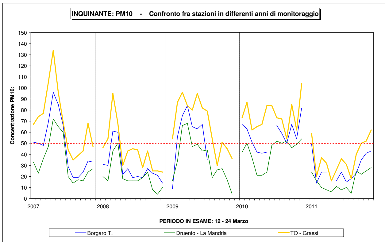
Figura 24 - Particolato sospeso PM 10 : confronto fra stazioni in differenti anni di monitoraggio
