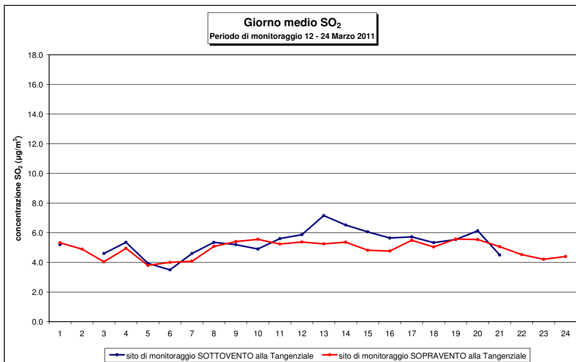
Figura 31 – Andamento del giorno medio di SO 2 per condizioni del sito di monitoraggio sopravvento e sottovento alla Tangenziale – con esclusione dei dati non rappresentativi
