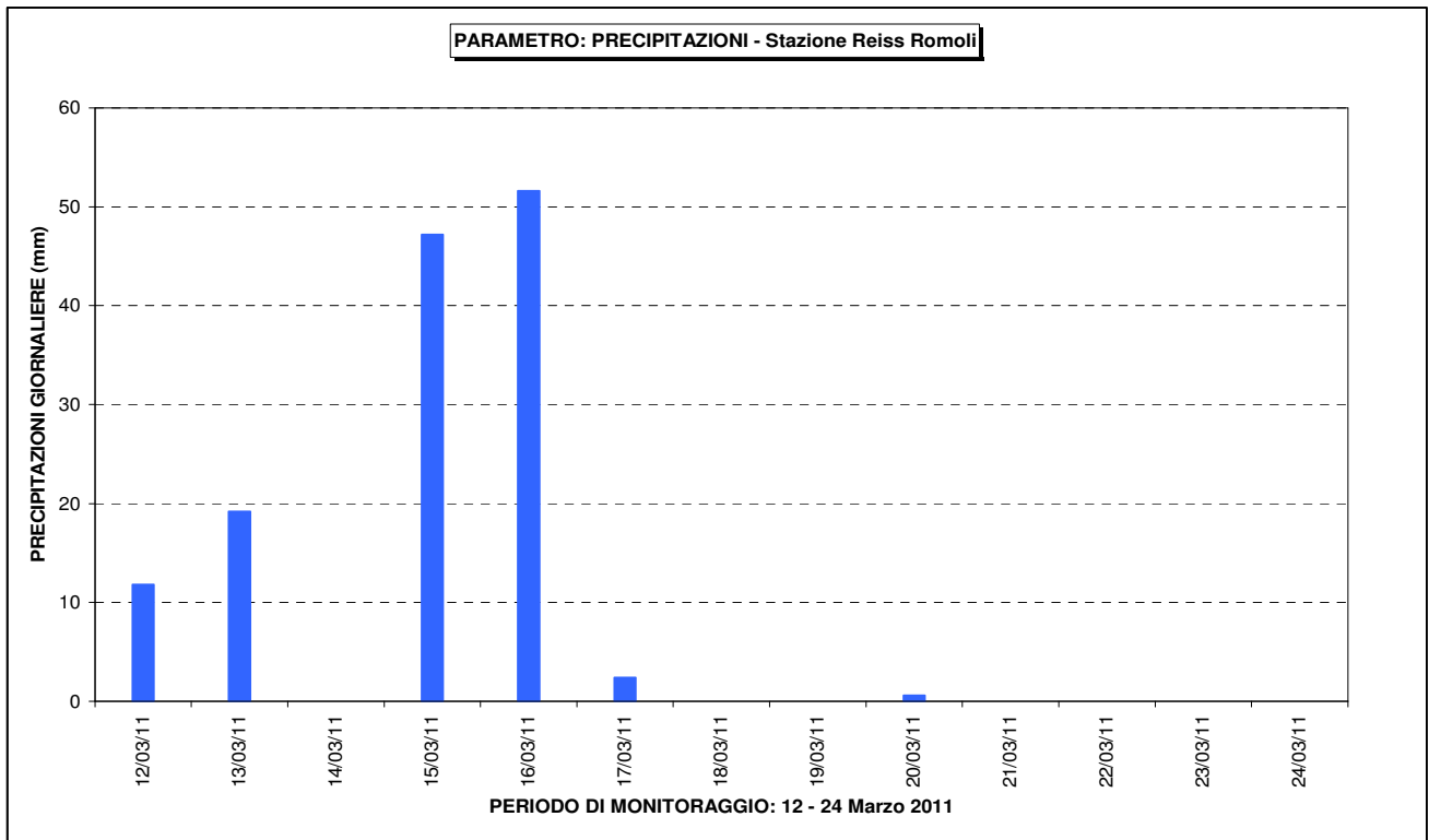
Figura 8 – Precipitazioni cumulate nel corso della campagna di monitoraggio
