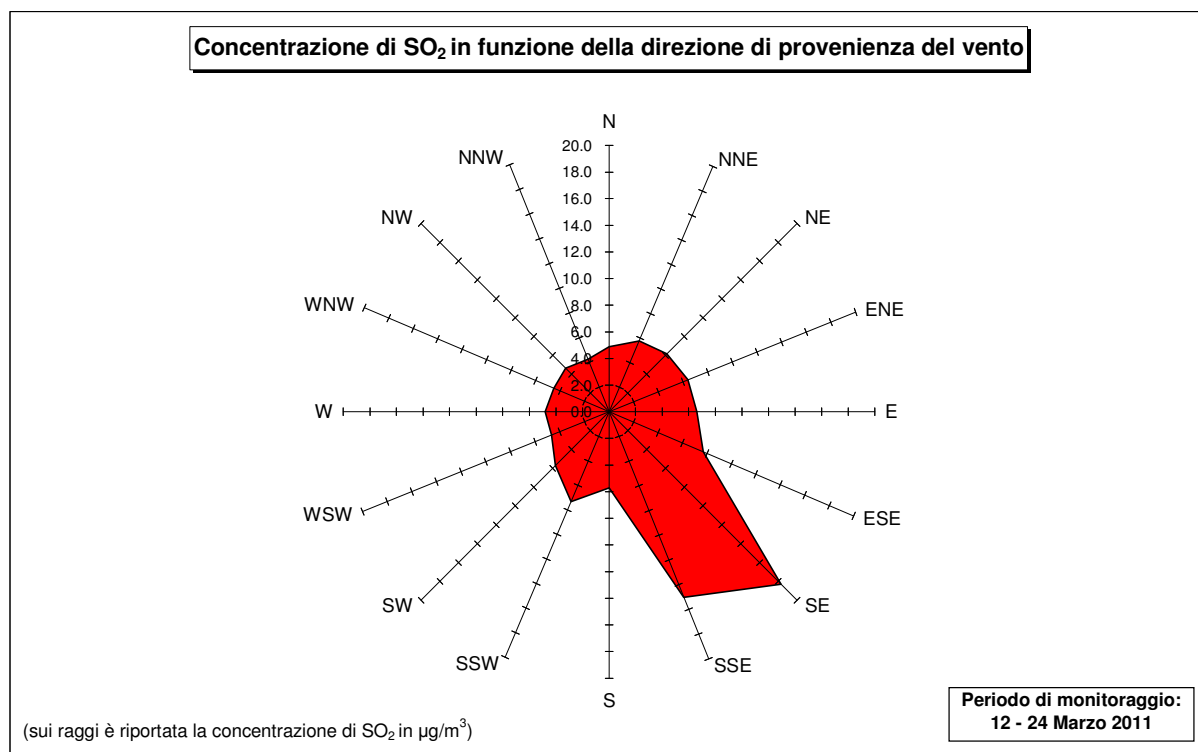
Figura 29 – Concentrazioni di SO 2 in funzione della direzione di provenienza del vento nel corso della campagna di monitoraggio nel Comune di Collegno
