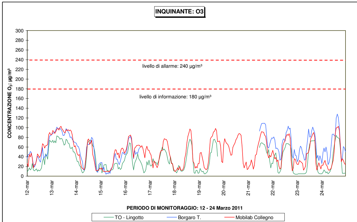
Figura 25 – O 3 : andamento della concentrazione oraria e confronto con i limiti di legge
