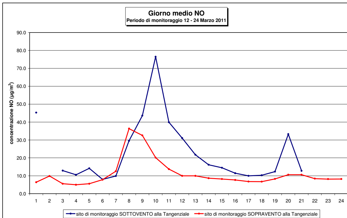
Figura 28 – Andamento del giorno medio di NO per condizioni del sito di monitoraggio sopravento e sottovento alla Tangenziale
