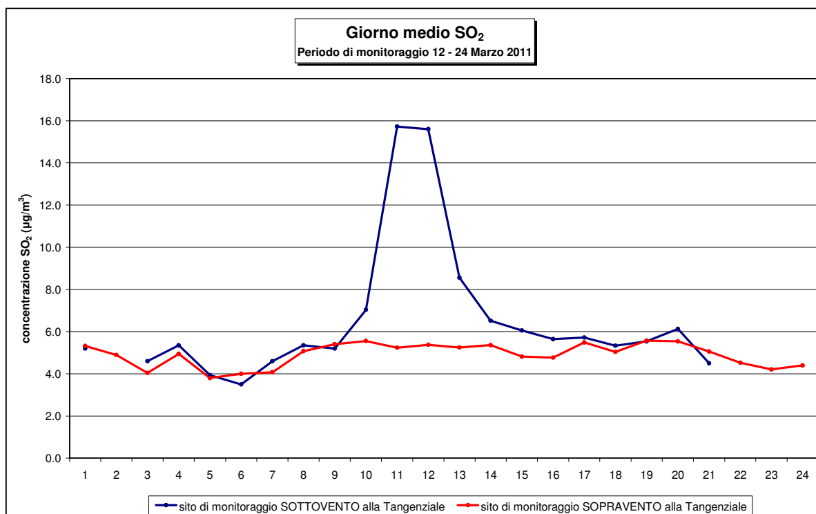
Figura 30 – Andamento del giorno medio di SO 2 per condizioni del sito di monitoraggio sopravvento e sottovento alla Tangenziale
