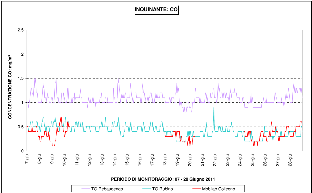
Figura 15 – CO: andamento della concentrazione oraria nel corso della campagna di monitoraggio e confronto con le stazioni fisse di Torino-Rebaudengo e Torino-Rubino
