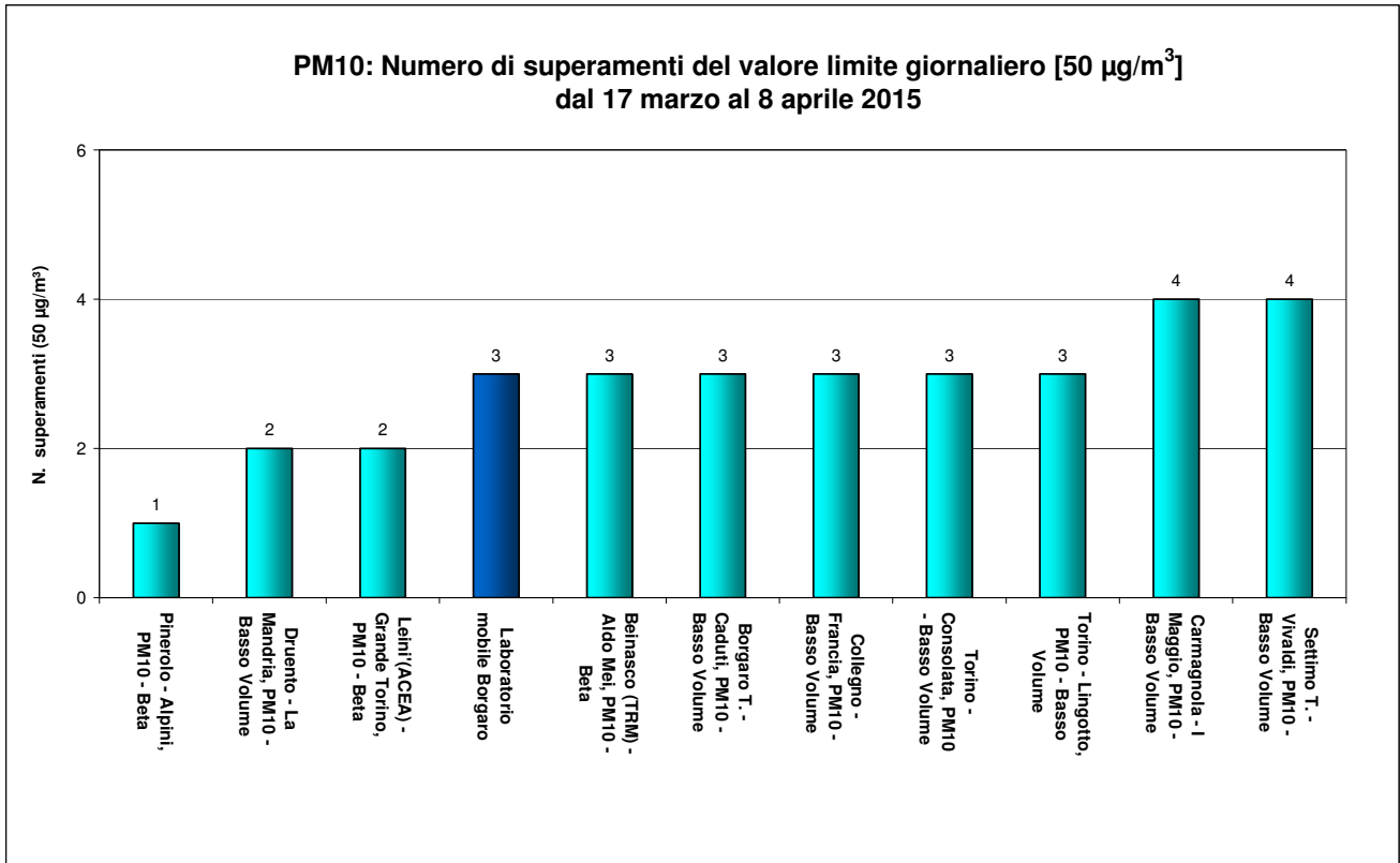
Figura 26: Particolato sospeso PM10 - numero di superamenti del valore limite giornaliero in provincia di Torino nel corso della prima campagna.
