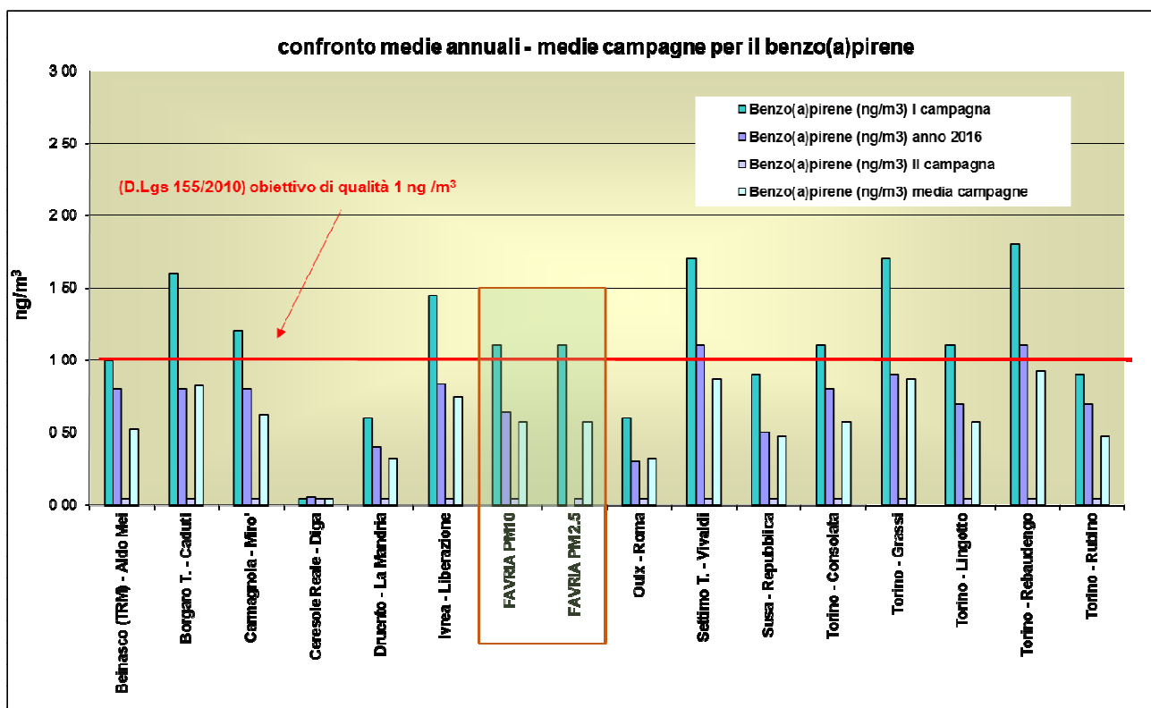
Figura 35 - Benzo(a)pirene confronto della media campagna invernale e primaverile con media anno 2016 nella provincia di Torino
