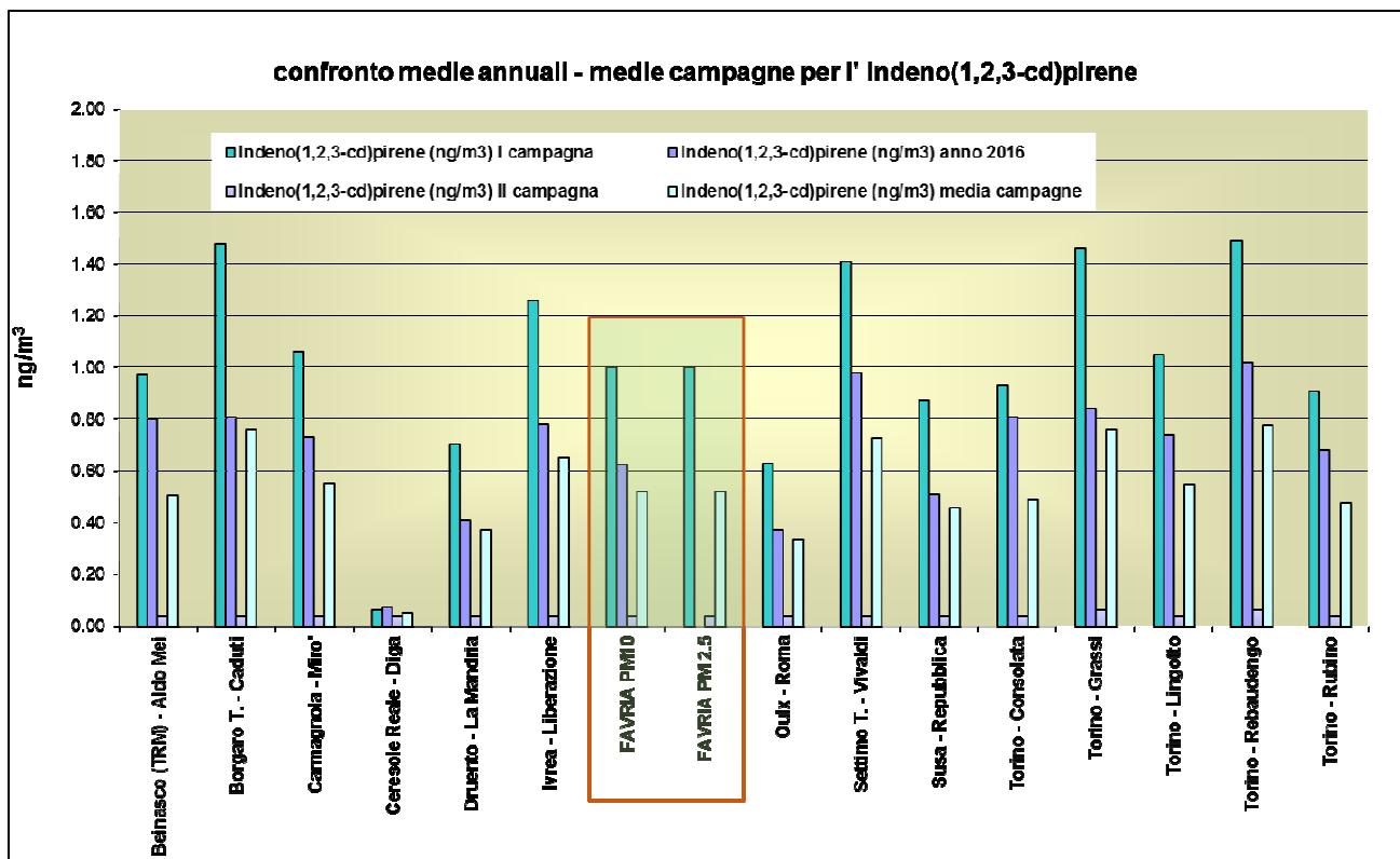
Figura 36 - Indeno(1, 2, 3-cd)pirene confronto della media campagna invernale e primaverile con media anno 2016 nella provincia di Torino
