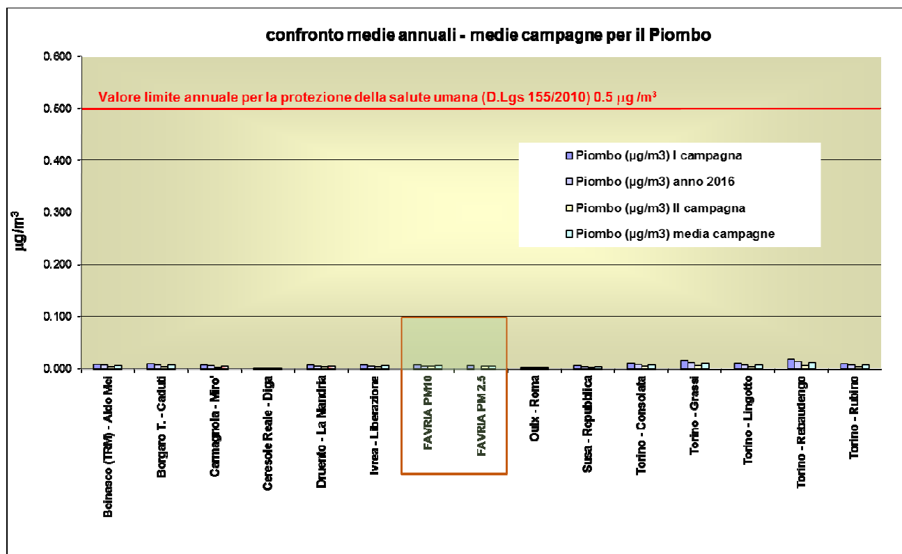
Figura 40 - Piombo confronto della media campagna invernale e primaverile con media anno 2016 nella provincia di Torino
