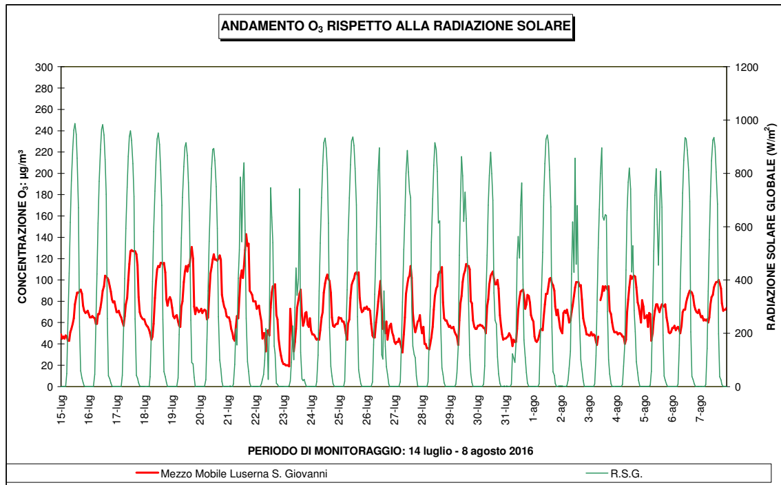
Figura 35: O 3 - andamento della concentrazione oraria e confronto con la radiazione solare globale
