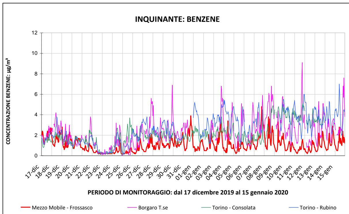
Figura 4: andamento Benzene a Frossasco – via Don Rinaldo Asvisio 4 durante la prima campagna di monitoraggio
