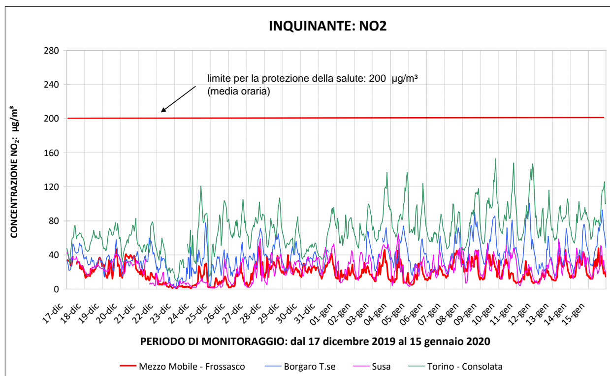
Figura 3: andamento NO 2 a Frossasco – durante la prima campagna di monitoraggio.
