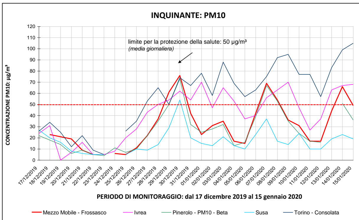
Figura 5: Andamento PM 10 a Frossasco – via Don Rinaldo Asvisio 4 durante campagna invernale
