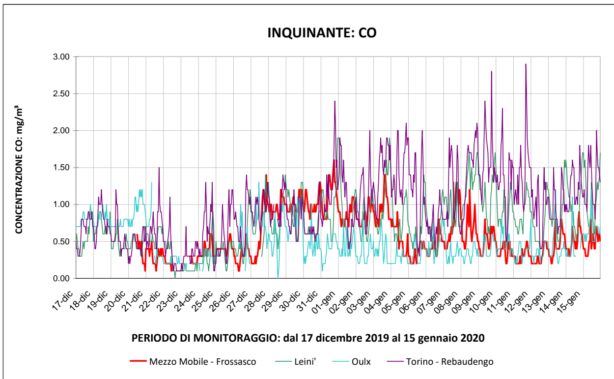
Figura 10 andamento CO a Frossasco – via Don Rinaldo Asvisio 4 durante la campagna invernale
