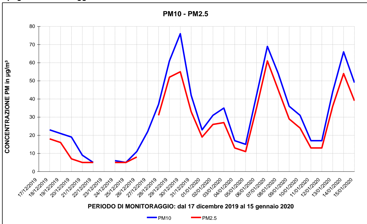
Figura 7: andamento PM10 e PM2.5 a Frossasco – Via Don Rinaldo Asvisio 4 durante la prima campagna di monitoraggio
