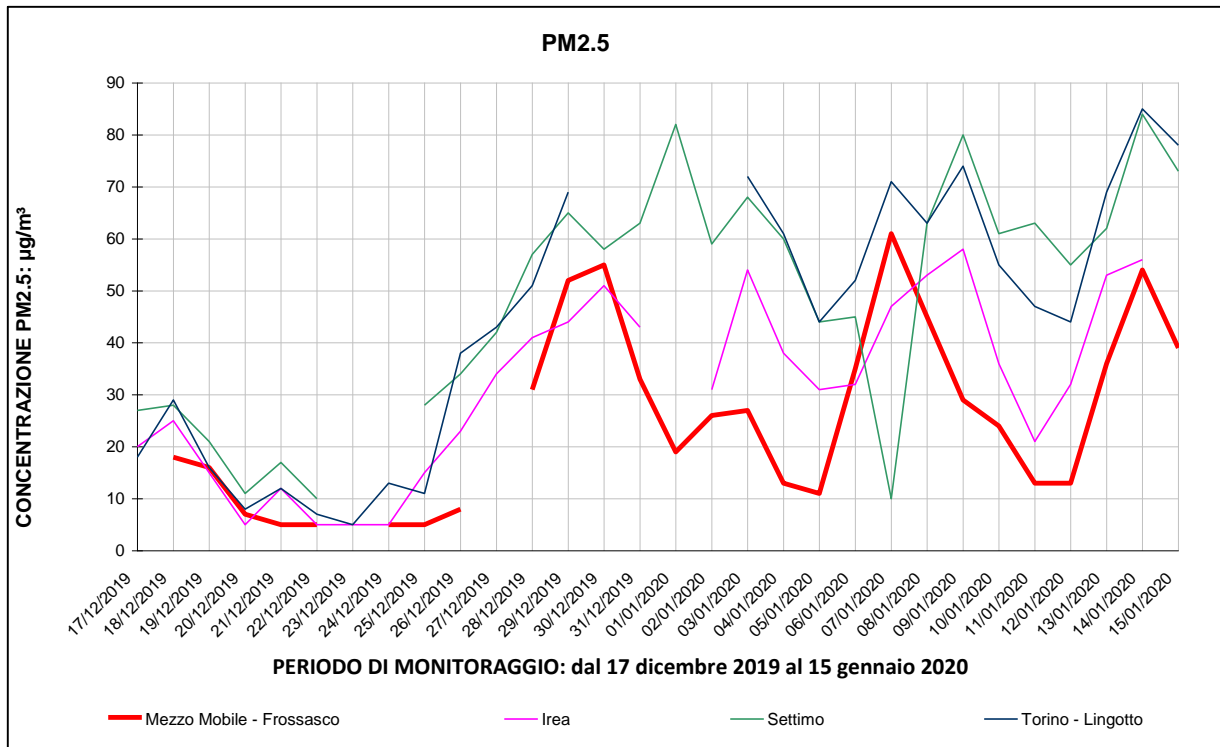
Figura 6: Andamento PM2.5 a Frossasco – Via Don Rinaldo Asvisio 4 durante la prima campagna di monitoraggio
