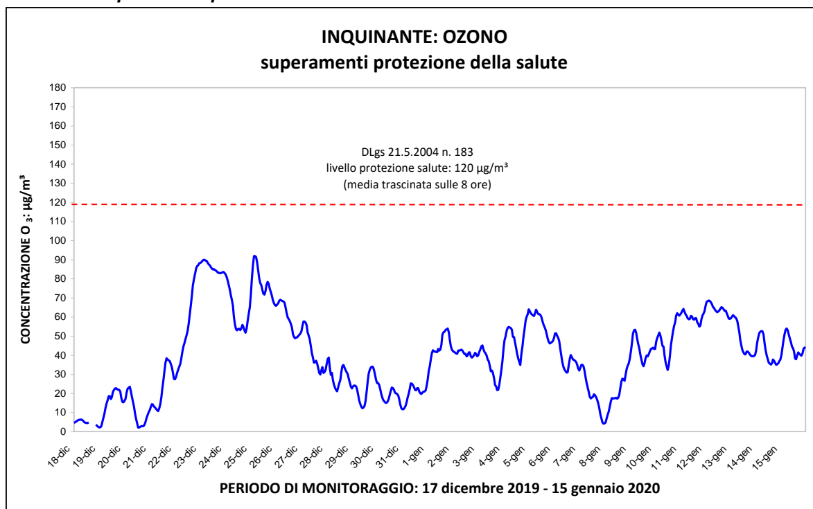
Figura 9: O 3 - superamenti protezione della salute umana
