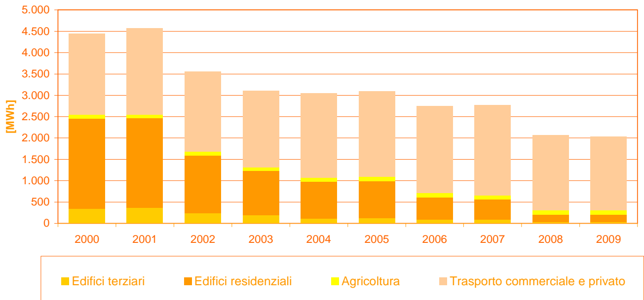
Grafico 21 – Consumo di gasolio per settore
