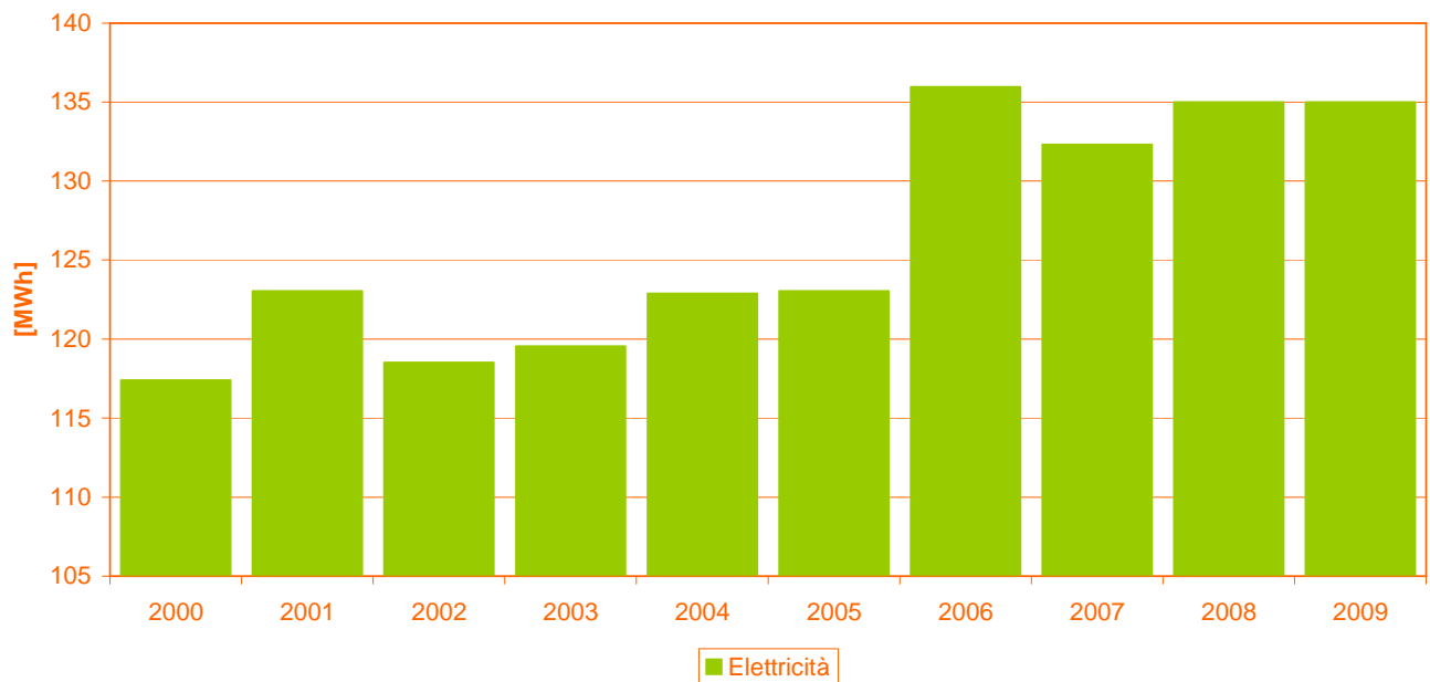
Grafico 29 - Consumi energetici dell'illuminazione pubblica
