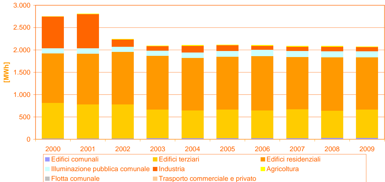
Grafico 16 – Consumo di elettricità per settore
