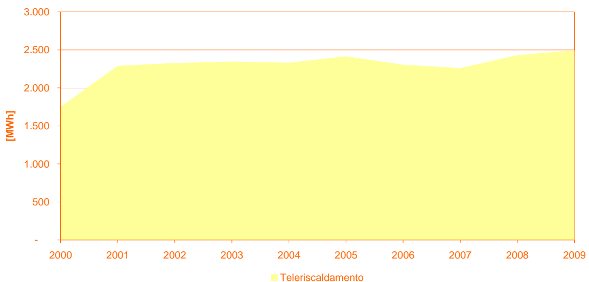
Grafico 39 – La produzione locale di energia termica nel Comune di Pomaretto dal 2000 al 2009
