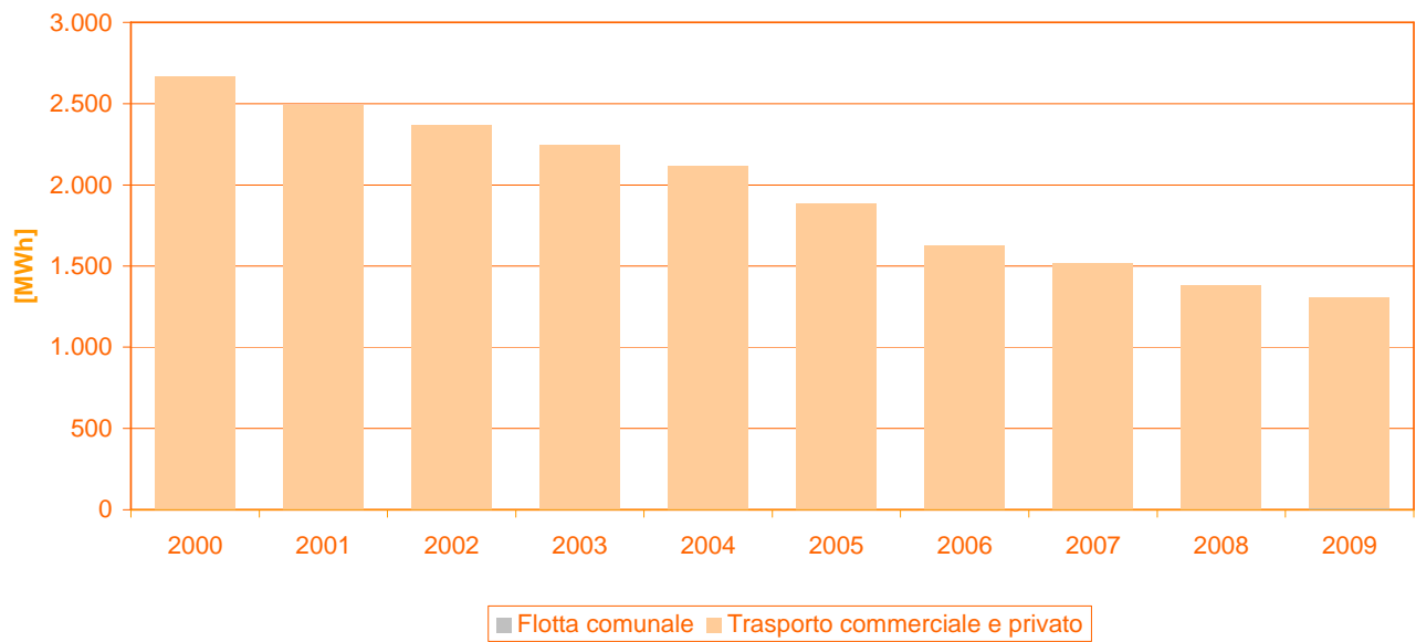
Grafico 22 – Consumo di benzina per settore
