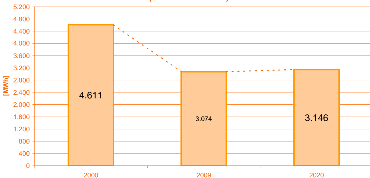
Grafico 56 – L’evoluzione dei consumi di energia per trazione nel settore dei trasporti (scenario Business as usual)
