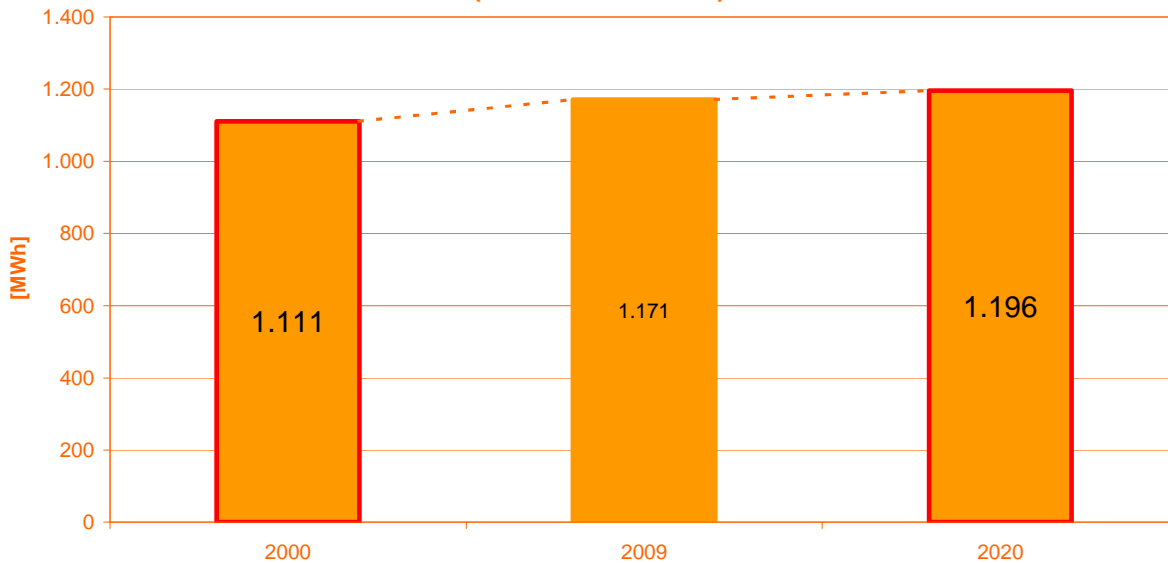
Grafico 53 – L'evoluzione dei consumi di energia elettrica negli edifici residenziali (scenario Business as usual)
