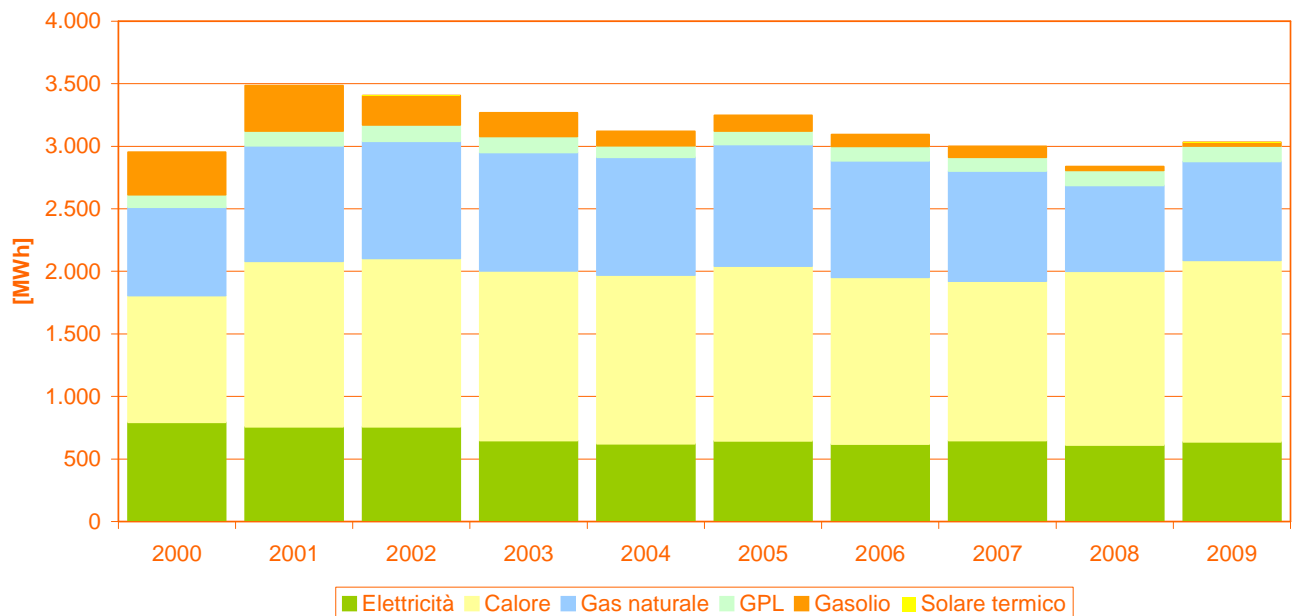
Grafico 26 - Consumi energetici del settore terziario
