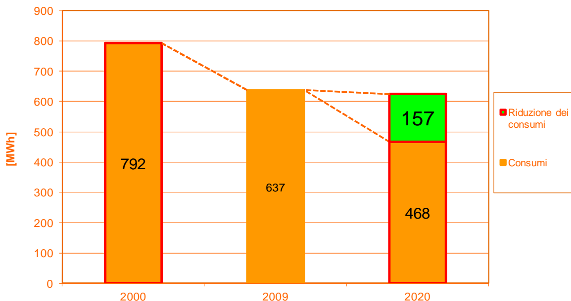
Evoluzione dei consumi di energia elettrica negli edifici terziari (attuazione del PAES)
