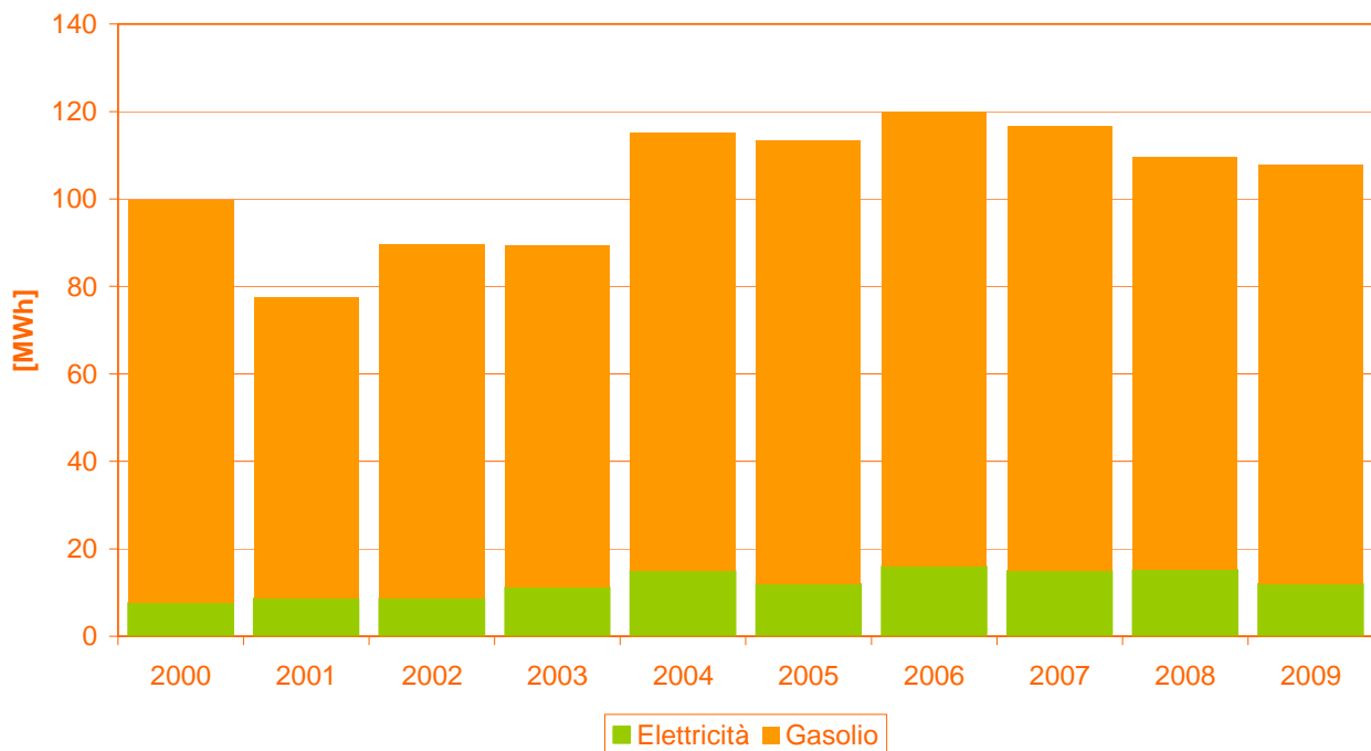
Grafico 36 - Consumi energetici del settore agricolo
