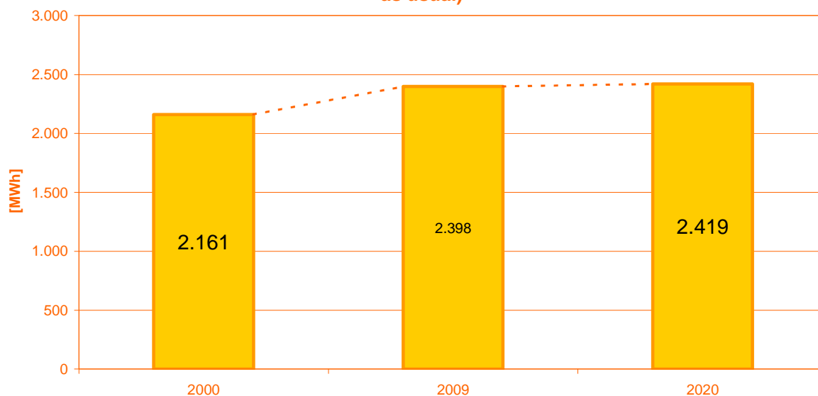
Grafico 54 – L'evoluzione dei consumi di energia termica negli edifici terziari (scenario Business as usual)
