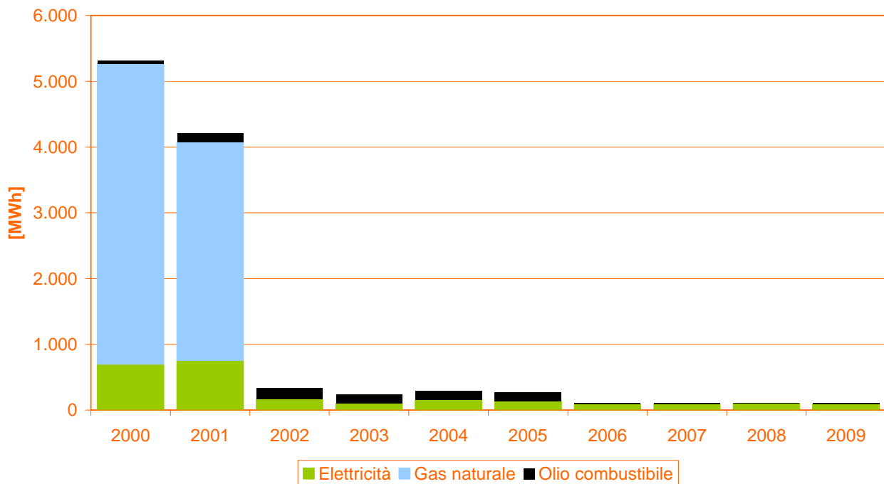
Grafico 34 – Consumi energetici nel settore industriale
