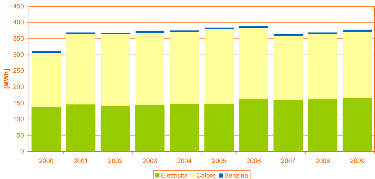
Grafico 28 - Consumi energetici del settore pubblico
