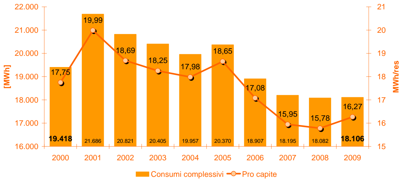
Grafico 15 – Consumi energetici complessivi e pro capite (industria ed agricoltura esclusi)
