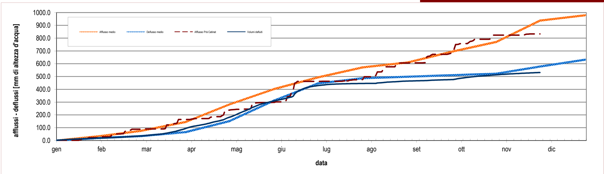
Diagramma cumulato degli afflussi e dei deflussi da inizio anno, espressi in mm di altezza d'acqua rapportati all'intera superficie del bacino idrografico contribuyente. I dati dell'anno in corso sono valori puntuali misurati da CHSPI e dal pluviometro di riferimento. L'afflusso medio di pioggia è relativo all'intero bacino (1995-2014); il deflusso medio è dato dalla media delle portate mensili misurate su CHSPI dal 2009 in poi.
