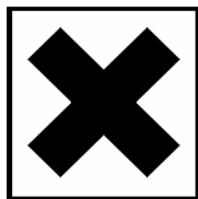
Xi - Irritante
