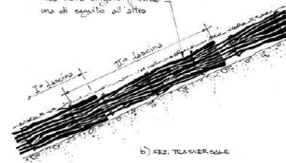
Posa in opera delle fascine
